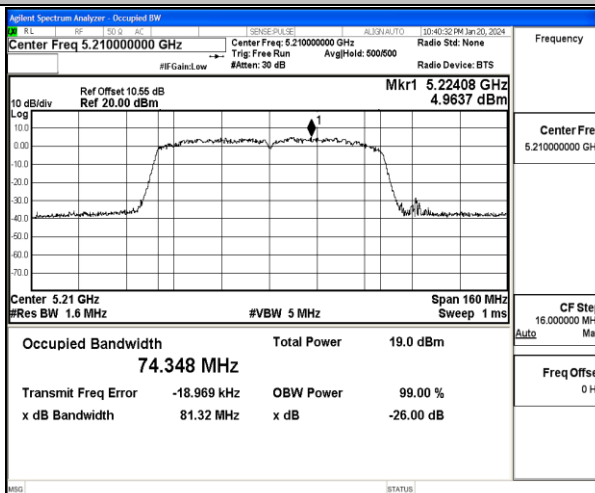
11AC80MIMO-Ant1-5210
