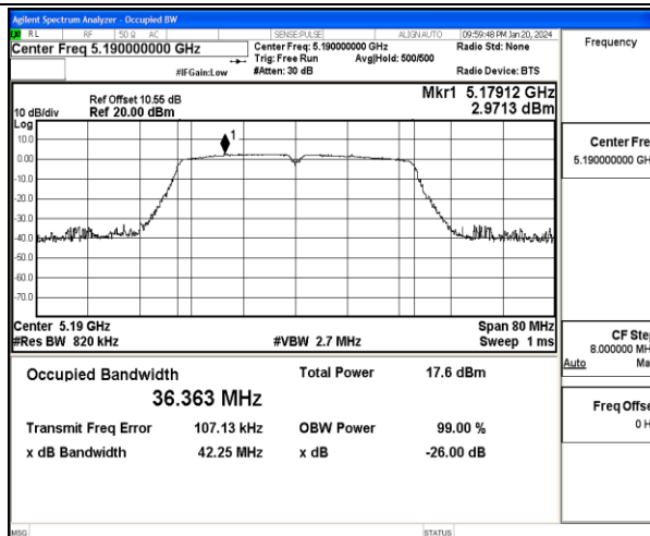
11N40MIMO-Ant1-5190
