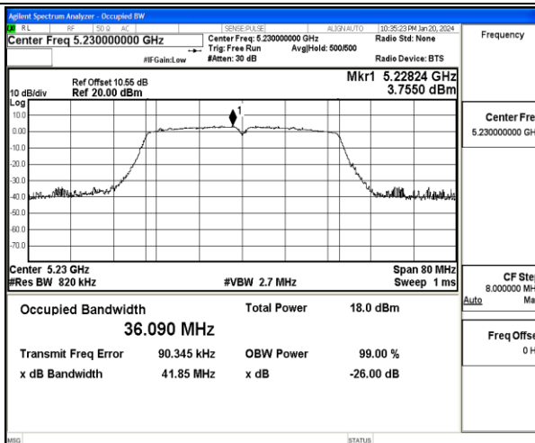
11AC40MIMO-Ant1-5230
