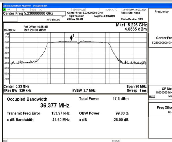
11N40MIMO-Ant1-5230
