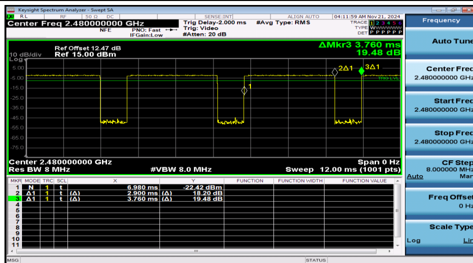
NTNV-2DH5-Ant1-2480
