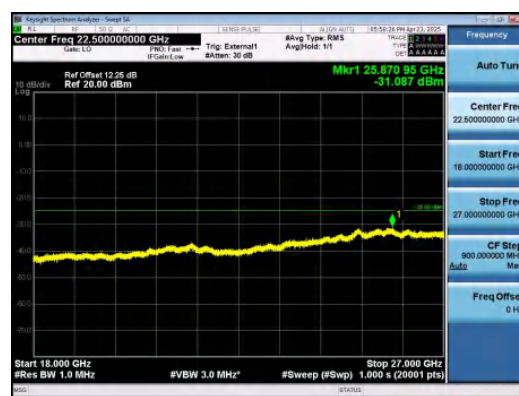
Band38-15MHz-16QAM-37825-1RB#0-18000~27000-PASS
