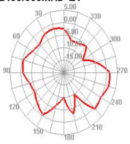
2450.000MHz E1
