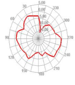
2500.000MHz E1
