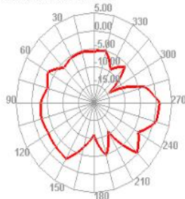
2400.000MHz E1
