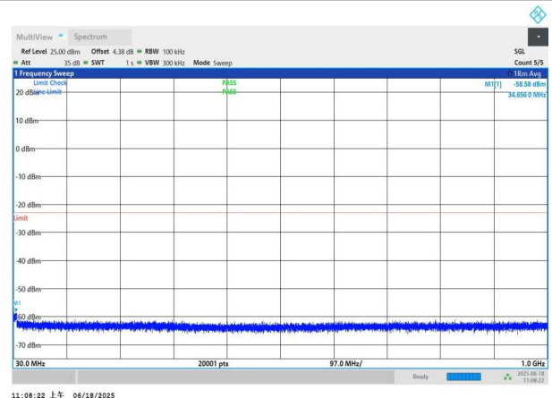
NTNV-n77(3700-3980)-PC3-30-20-M-DFT-QPSK-Edge_1RB_Left -30-1000-PASS
