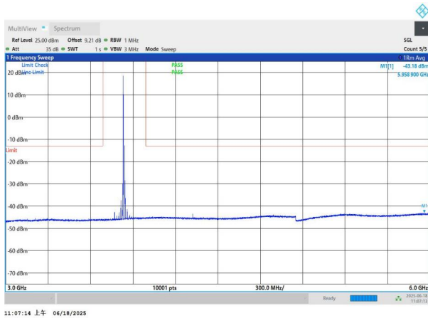
NTNV-n77(3700-3980)-PC3-30-20-M-DFT-BPSK-Edge_1RB_Left -3000-6000-PASS
