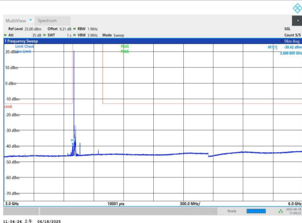
NTNV-n77(3700-3980)-PC3-30-20-L-DFT-BPSK-Edge_1RB_Left- 3000-6000-PASS
