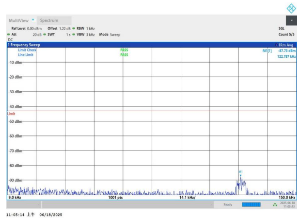
NTNV-n77(3700-3980)-PC3-30-20-L-DFT-QPSK-Edge_1RB_Left- 0.009-0.15-PASS
