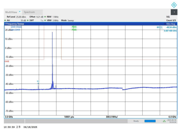
NTNV-n77(3700-3980)-PC3-30-15-M-DFT-QPSK-Edge_1RB_Left -3000-6000-PASS
