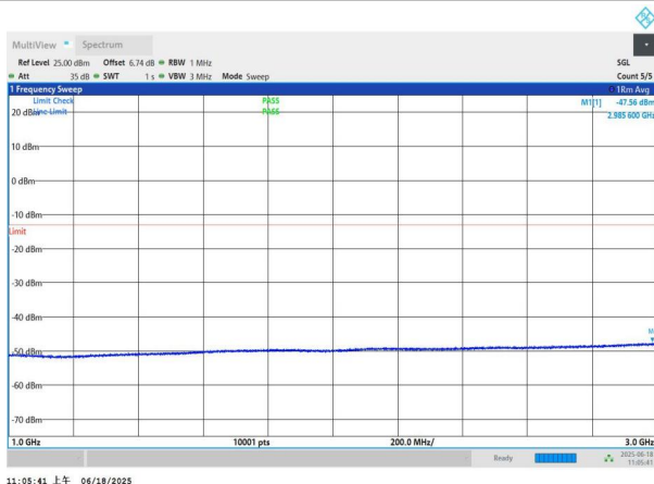
NTNV-n77(3700-3980)-PC3-30-20-L-DFT-QPSK-Edge_1RB_Left- 1000-3000-PASS
