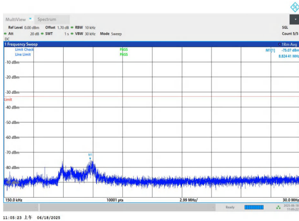
NTNV-n77(3700-3980)-PC3-30-20-L-DFT-QPSK-Edge_1RB_Left- 0.15-30-PASS
