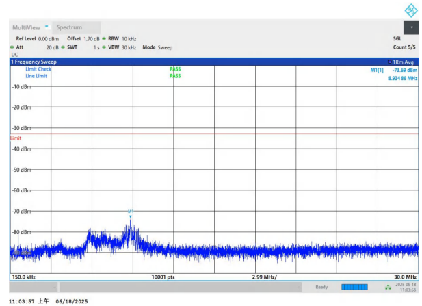
NTNV-n77(3700-3980)-PC3-30-20-L-DFT-BPSK-Edge_1RB_Left- 0.15-30-PASS
