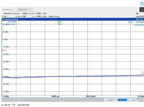
NTNV-n77(3700-3980)-PC3-30-20-M-DFT-QPSK-Edge_1RB_Left -1000-3000-PASS
