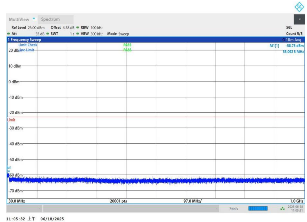
NTNV-n77(3700-3980)-PC3-30-20-L-DFT-QPSK-Edge_1RB_Left- 30-1000-PASS
