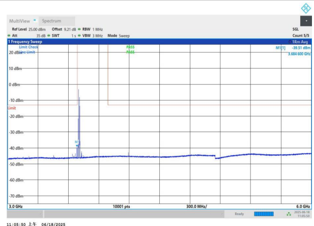
NTNV-n77(3700-3980)-PC3-30-20-L-DFT-QPSK-Edge_1RB_Left- 3000-6000-PASS
