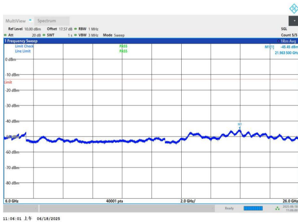
NTNV-n77(3700-3980)-PC3-30-20-L-DFT-QPSK-Edge_1RB_Left- 6000-26000-PASS
