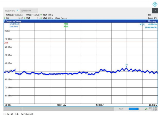
NTNV-n77(3700-3980)-PC3-30-20-L-DFT-BPSK-Edge_1RB_Left- 6000-26000-PASS
