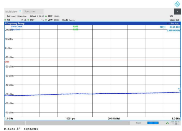
NTNV-n77(3700-3980)-PC3-30-20-L-DFT-BPSK-Edge_1RB_Left- 1000-3000-PASS
