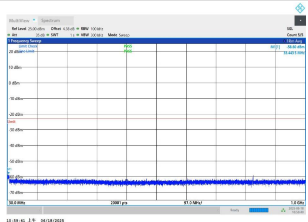
NTNV-n77(3700-3980)-PC3-30-15-M-DFT-QPSK-Edge_1RB_Left -30-1000-PASS
