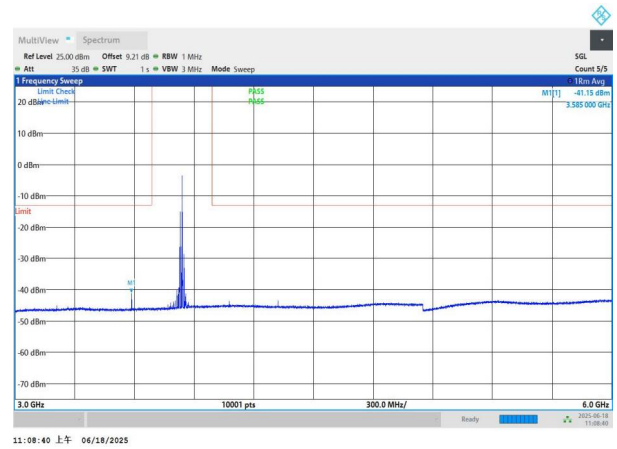
NTNV-n77(3700-3980)-PC3-30-20-M-DFT-QPSK-Edge_1RB_Left -3000-6000-PASS
