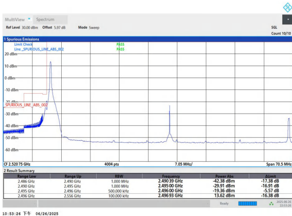
NTNV-n41-PC3-30-60-L-DFT-BPSK-Edge_1RB_Left-PASS
