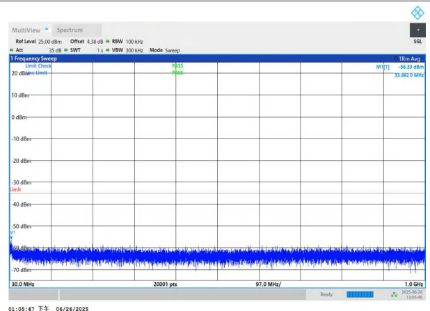
NTNV-n7-PC3-15-15-M-DFT-QPSK-Edge_1RB_Left-30-1000-PA SS
