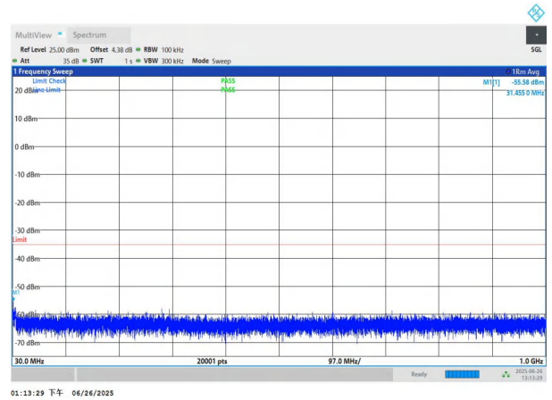
NTNV-n7-PC3-15-25-M-DFT-QPSK-Edge_1RB_Left-30-1000-PA SS
