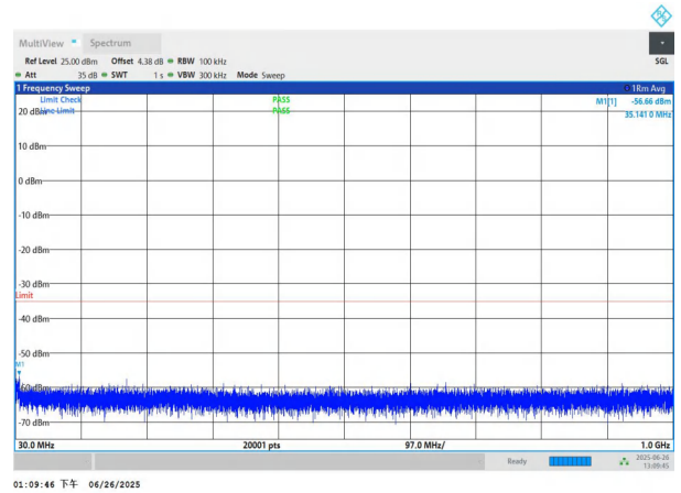
NTNV-n7-PC3-15-20-M-DFT-QPSK-Edge_1RB_Left-30-1000-PA SS
