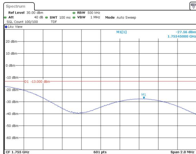
Band4-20MHz-QPSK-20300-1RB#99
