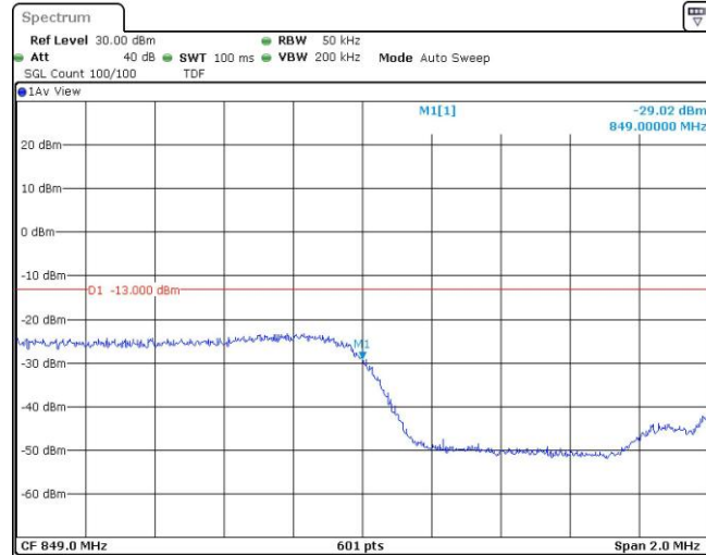
Band5-3MHz-QPSK-20635-1RB#14
