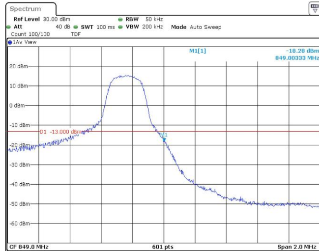
Band5-3MHz-QPSK-20635-15RB#0
