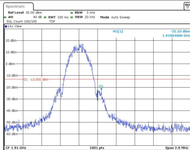
EGPRS1900-810-2
