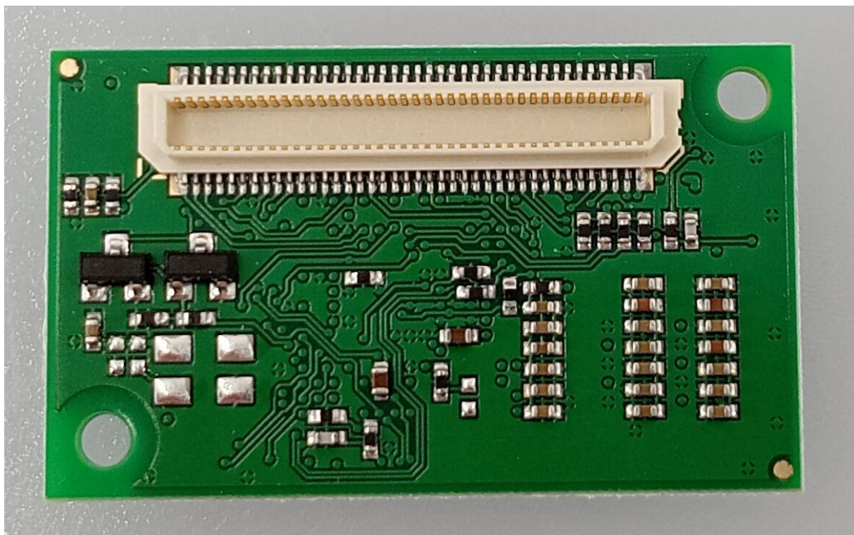
Figure 8 – SOM (back)
