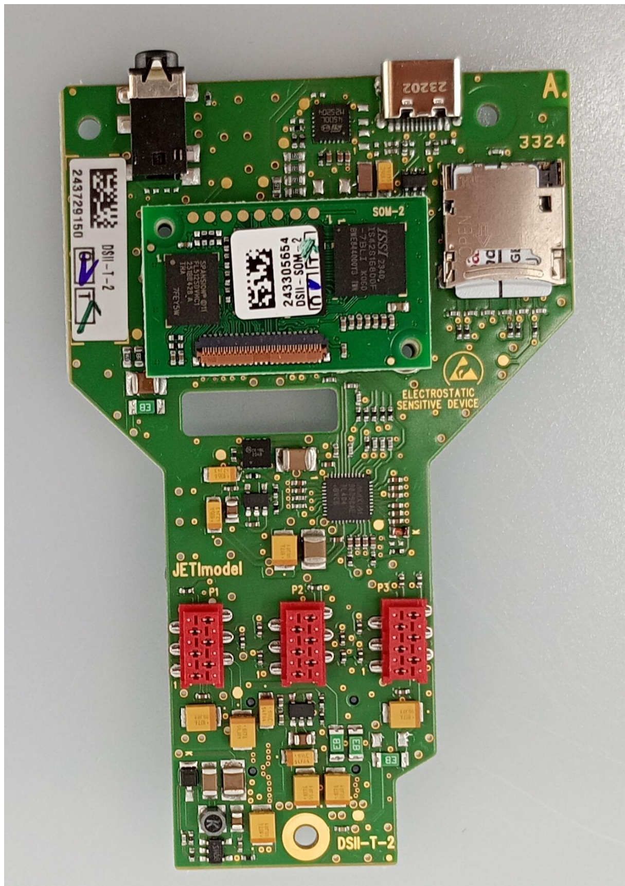
Figure 9 – DS24II-T + SOM
