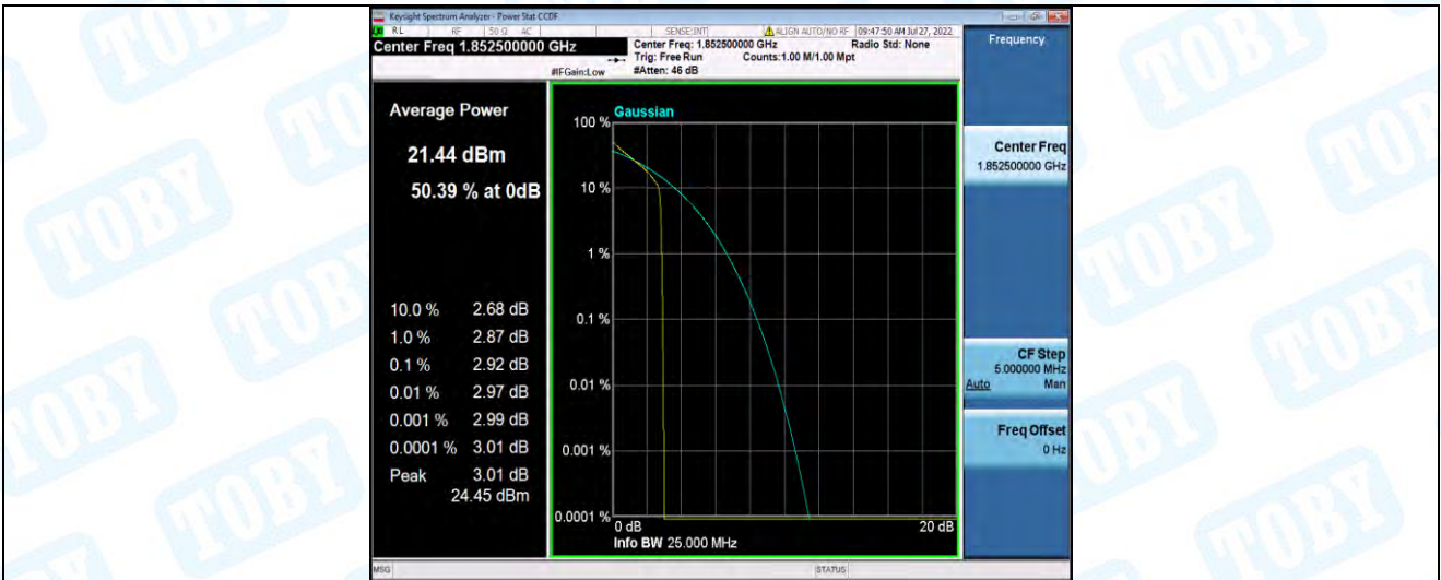
Band2-5MHz-QPSK-18625-25RB#0
