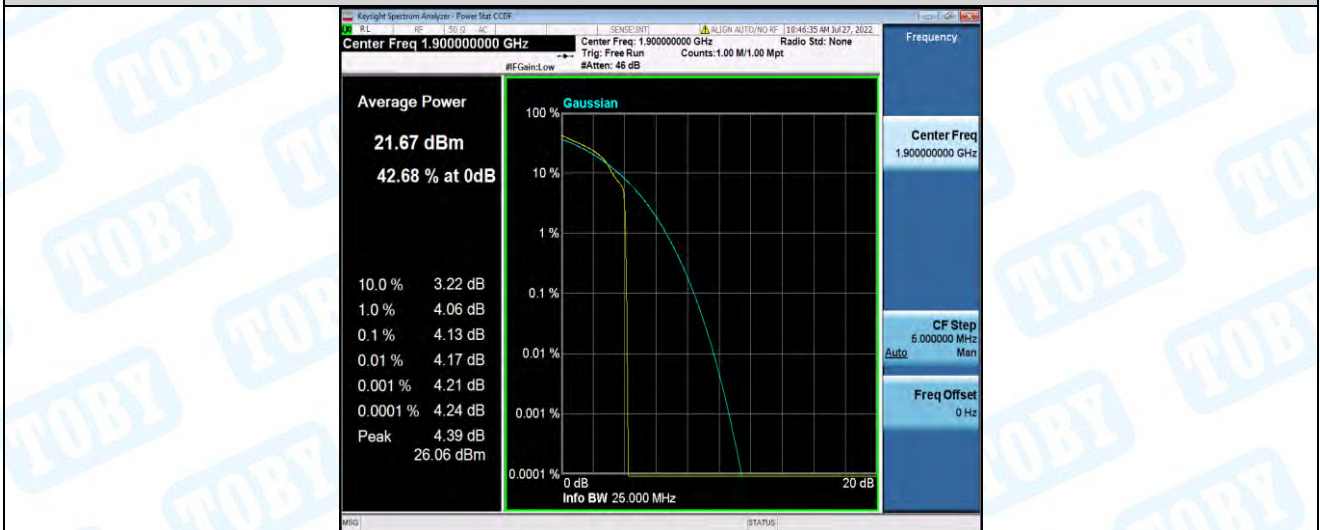
Band2-20MHz-16QAM-19100-100RB#0
