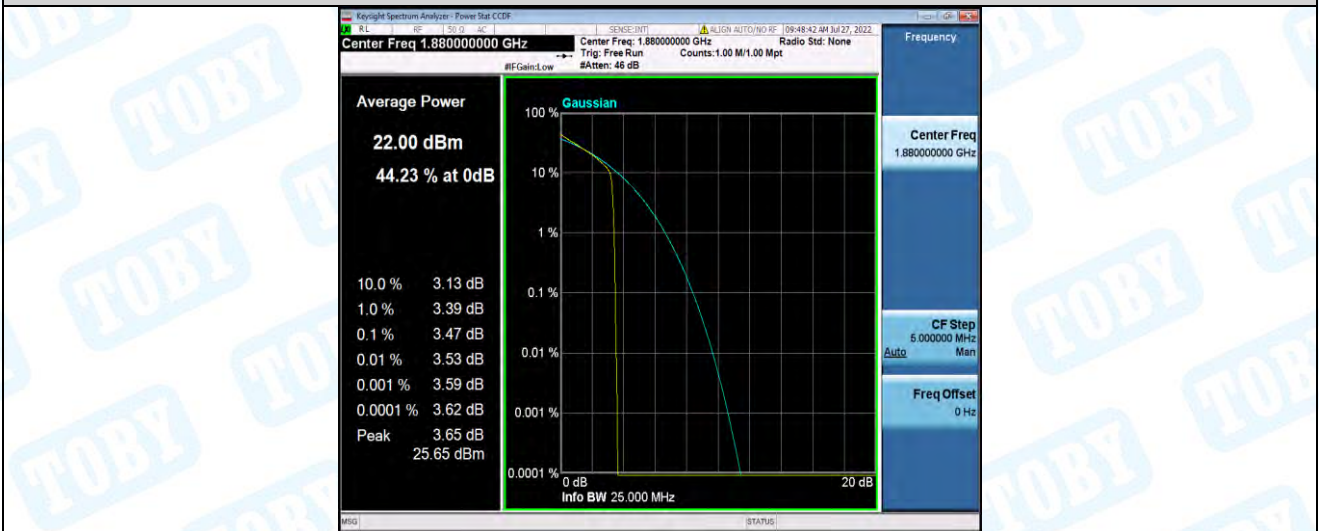
Band2-5MHz-QPSK-18900-25RB#0
