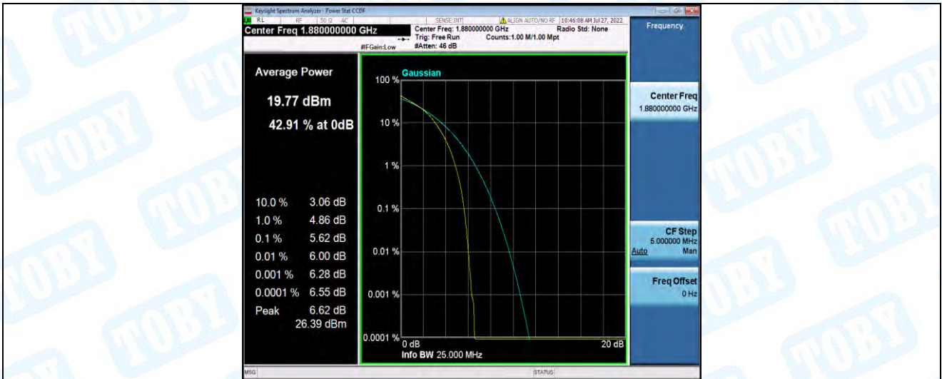
Band2-20MHz-16QAM-19100-1RB#0
