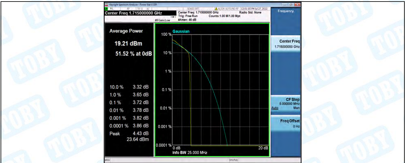
Band4-10MHz-QPSK-20000-50RB#0
