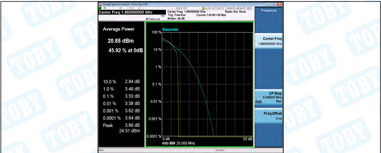
Band2-20MHz-16QAM-18700-100RB#0
