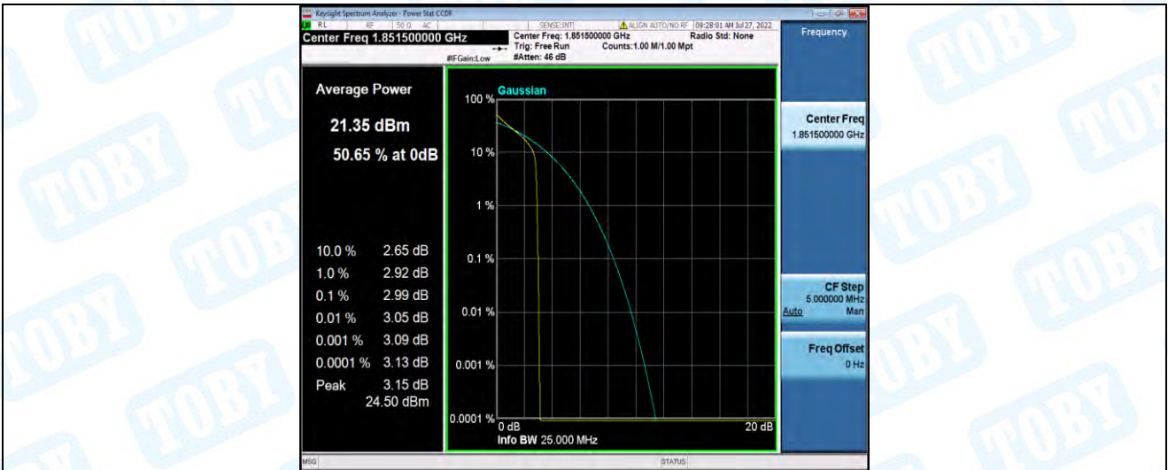
Band2-3MHz-QPSK-18615-15RB#0
