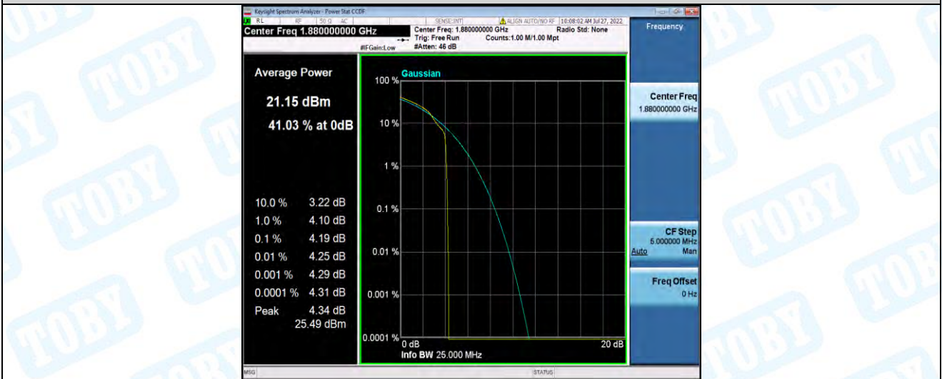
Band2-10MHz-16QAM-18900-50RB#0
