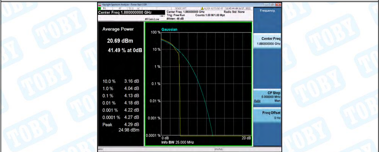
Band2-20MHz-16QAM-18900-100RB#0
