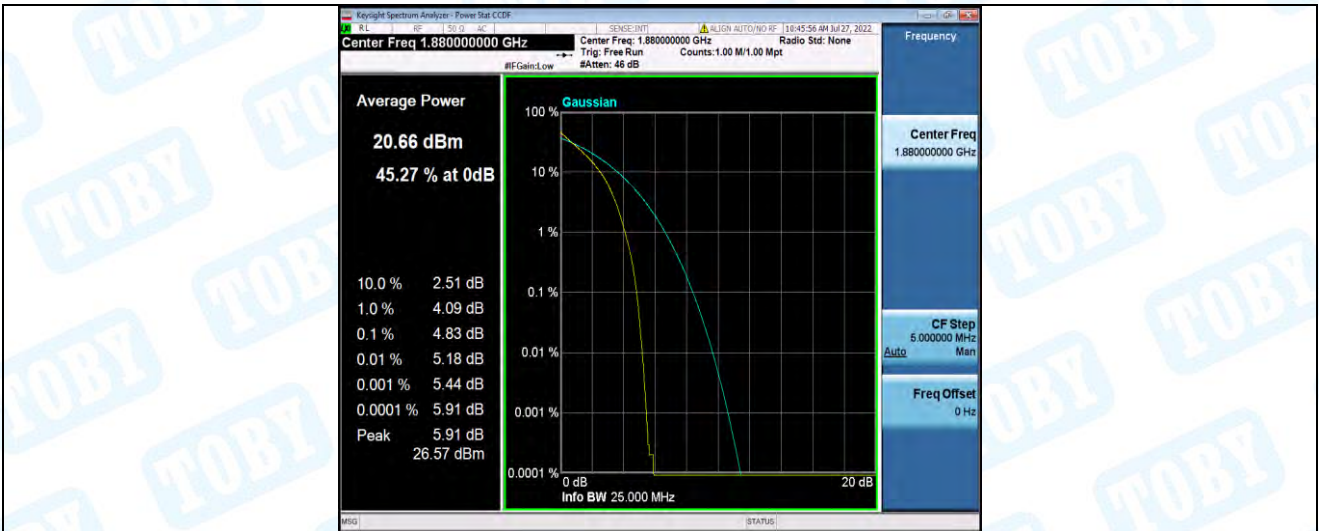
Band2-20MHz-QPSK-19100-1RB#0
