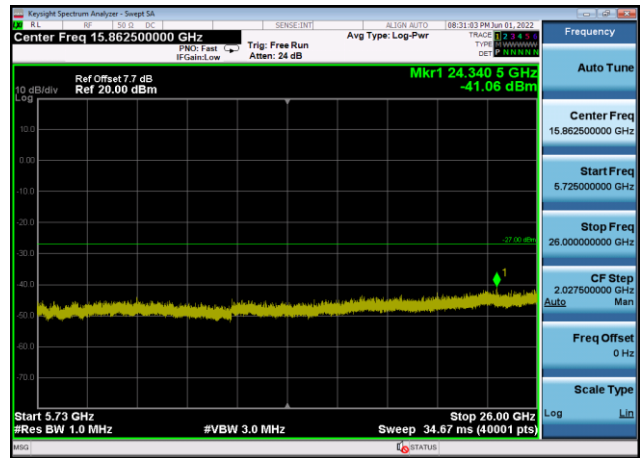
U-NII-2c ,Plot 3,5725MHz~26000MHz-802 .11ac(20MHz),5700MHz,Ant9
