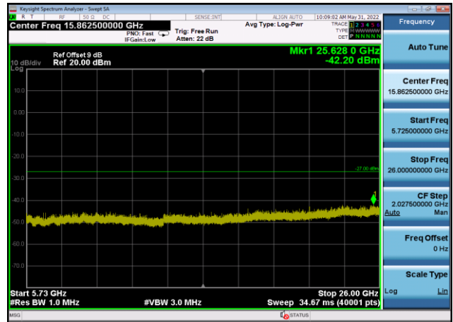
U-NII-2c ,Plot 3,5725MHz~26000MHz-802 .11ac(40MHz),5510MHz,Ant9
