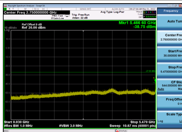
U-NII-2c ,Plot 2,30MHz~5470MHz-802.11 a(20MHz),5500MHz,Ant9
