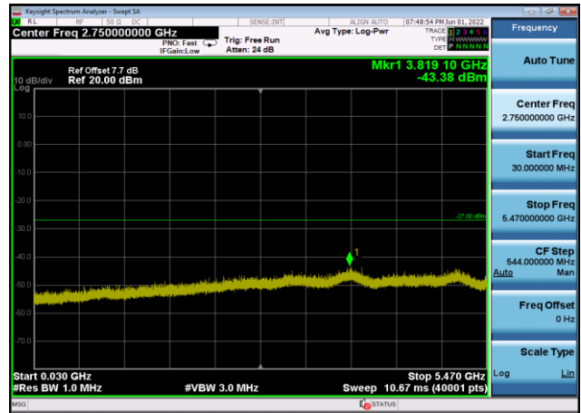
U-NII-2c ,Plot 2,30MHz~5470MHz-802.11 ax(40MHz),5670MHz,Ant8
