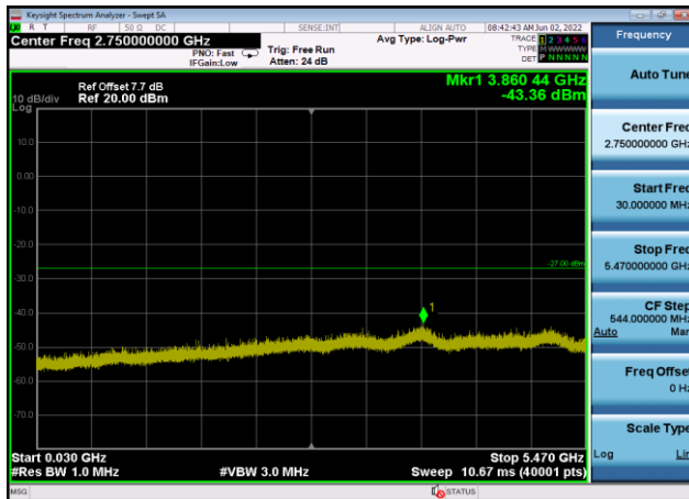
U-NII-2c ,Plot 2,30MHz~5470MHz-802.11 a(20MHz),5600MHz,Ant8
