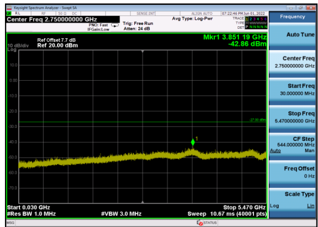
U-NII-2c ,Plot 2,30MHz~5470MHz-802.11 ax(160MHz),5570MHz,Ant8
