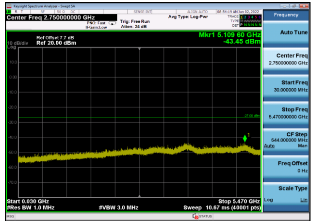
U-NII-2c ,Plot 2,30MHz~5470MHz-802.11 ax(20MHz),5700MHz,Ant8
