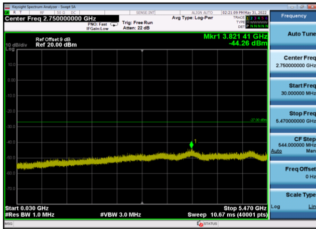
U-NII-2c ,Plot 2,30MHz~5470MHz-802.11 ax(80MHz),5610MHz,Ant9
