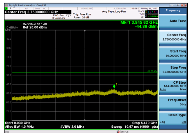
U-NII-2c ,Plot 2,30MHz~5470MHz-802.11 ac(160MHz),5570MHz,Ant9
