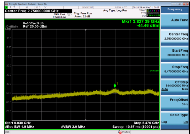
U-NII-2c ,Plot 2,30MHz~5470MHz-802.11 a(20MHz),5700MHz,Ant9
