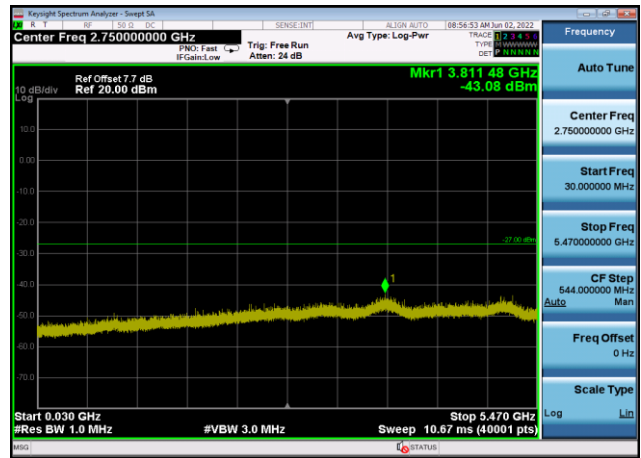
U-NII-2c ,Plot 2,30MHz~5470MHz-802.11 ax(20MHz),5600MHz,Ant8
