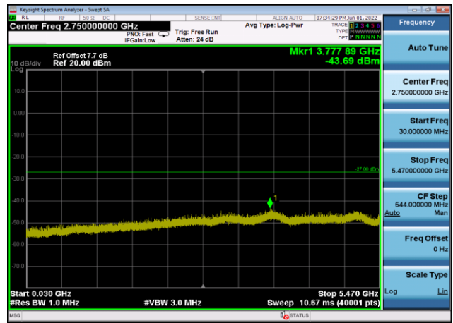
U-NII-2c ,Plot 2,30MHz~5470MHz-802.11 ac(80MHz),5610MHz,Ant8
