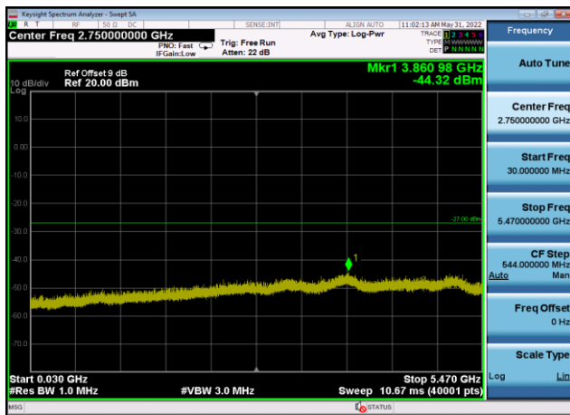
U-NII-2c ,Plot 2,30MHz~5470MHz-802.11 ax(40MHz),5670MHz,Ant9
