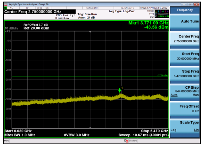
U-NII-2c ,Plot 2,30MHz~5470MHz-802.11 ax(80MHz),5610MHz,Ant8
