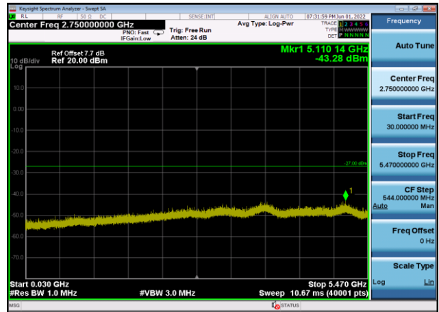
U-NII-2c ,Plot 2,30MHz~5470MHz-802.11 ax(160MHz),5570MHz,Ant8
