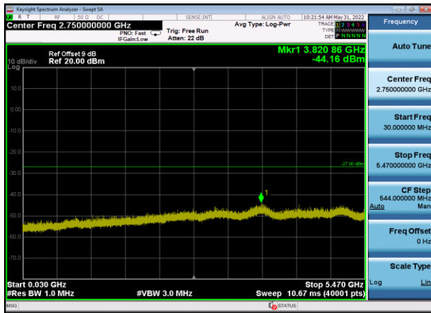
U-NII-2c ,Plot 2,30MHz~5470MHz-802.11 ax(20MHz),5600MHz,Ant9
