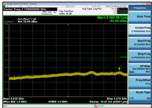
U-NII-2c ,Plot 2,30MHz~5470MHz-802.11 ax(20MHz),5700MHz,Ant8
