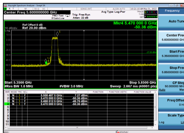
U-NII-2c ,Plot 1,Band Edge-802.11ax(2 0MHz),5600MHz,Ant9
