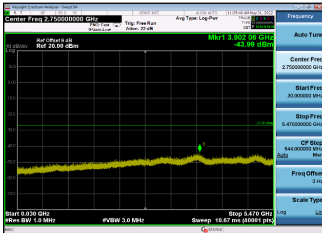
U-NII-2c ,Plot 2,30MHz~5470MHz-802.11 ac(40MHz),5590MHz,Ant9
