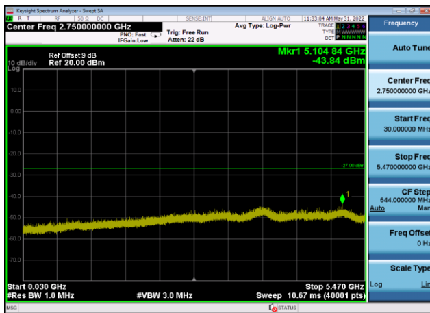
U-NII-2c ,Plot 2,30MHz~5470MHz-802.11 ac(40MHz),5670MHz,Ant9
