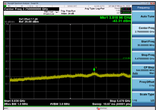
U-NII-2c ,Plot 2,30MHz~5470MHz-802.11 ac(40MHz),5590MHz,Ant8
