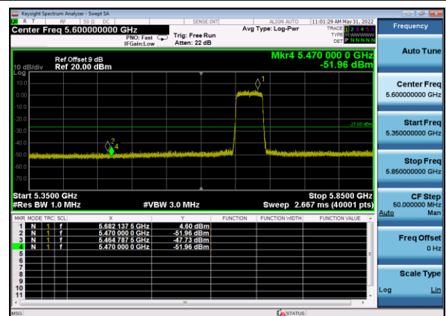
U-NII-2c ,Plot 1,Band Edge-802.11ax(4 0MHz),5670MHz,Ant9
