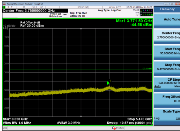
U-NII-2c ,Plot 2,30MHz~5470MHz-802.11 ax(40MHz),5590MHz,Ant9
