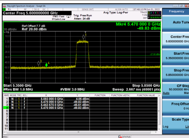
U-NII-2c ,Plot 1,Band Edge-802.11ax(4 0MHz),5590MHz,Ant8
