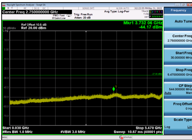
U-NII-2c ,Plot 2,30MHz~5470MHz-802.11 ax(160MHz),5570MHz,Ant9
