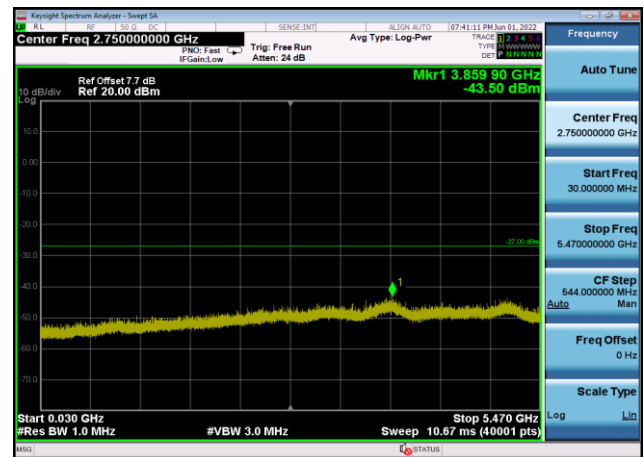
U-NII-2c ,Plot 2,30MHz~5470MHz-802.11 ac(40MHz),5670MHz,Ant8
