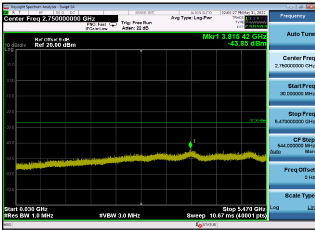
U-NII-2c ,Plot 2,30MHz~5470MHz-802.11 ac(80MHz),5610MHz,Ant9
