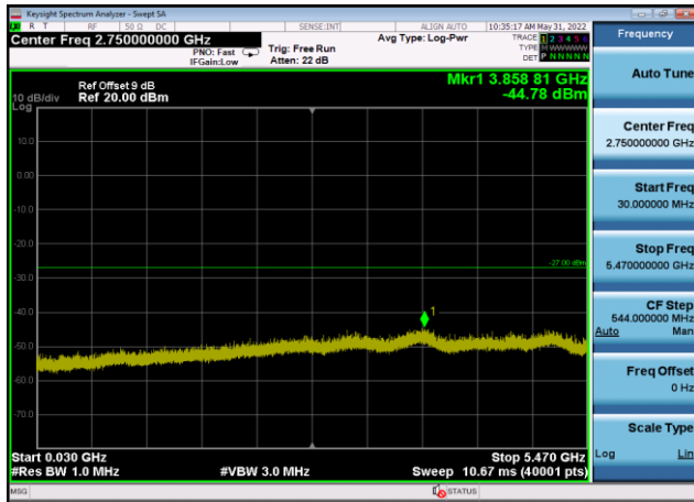
U-NII-2c ,Plot 2,30MHz~5470MHz-802.11 ax(20MHz),5700MHz,Ant9
