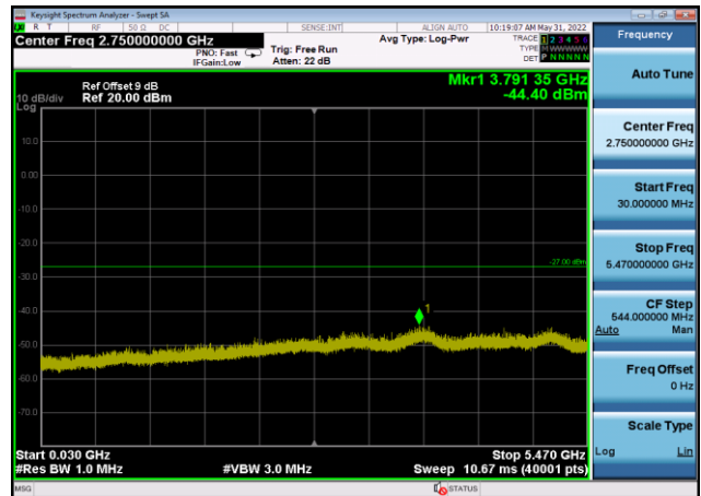
U-NII-2c ,Plot 2,30MHz~5470MHz-802.11 ac(20MHz),5600MHz,Ant9
