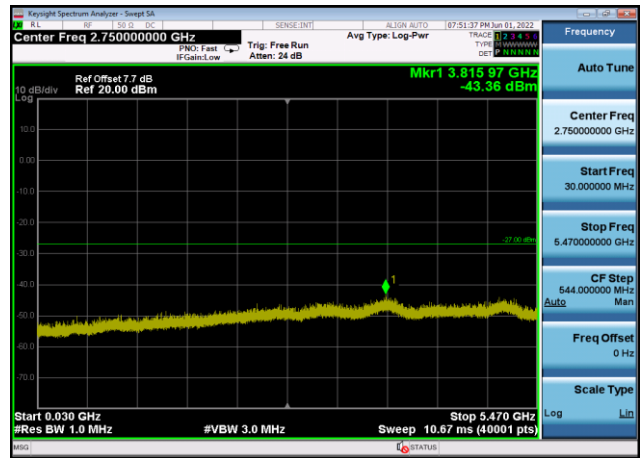
U-NII-2c ,Plot 2,30MHz~5470MHz-802.11 ax(40MHz),5590MHz,Ant8
