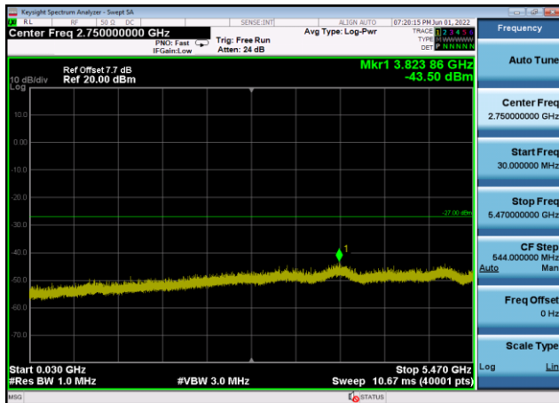
U-NII-2c ,Plot 2,30MHz~5470MHz-802.11 ac(20MHz),5500MHz,Ant8
