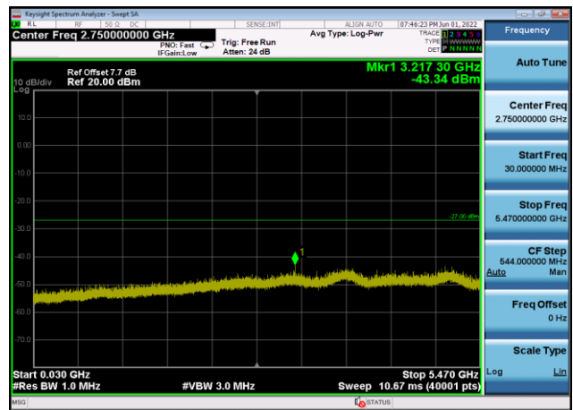
U-NII-2c ,Plot 2,30MHz~5470MHz-802.11 ax(40MHz),5670MHz,Ant8
