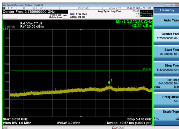
U-NII-2c ,Plot 2,30MHz~5470MHz-802.11 a(20MHz),5700MHz,Ant8
