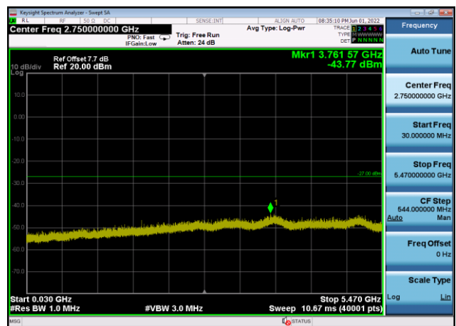
U-NII-2c ,Plot 2,30MHz~5470MHz-802.11 ac(20MHz),5700MHz,Ant8
