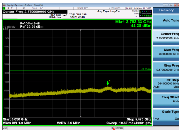
U-NII-2c ,Plot 2,30MHz~5470MHz-802.11 ac(20MHz),5700MHz,Ant9
