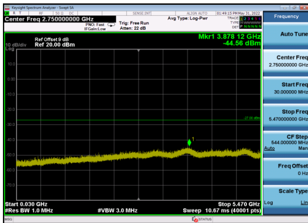
U-NII-2c ,Plot 2,30MHz~5470MHz-802.11 n(40MHz),5670MHz,Ant9
