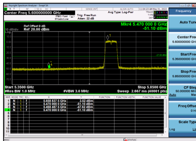
U-NII-2c ,Plot 1,Band Edge-802.11ac(4 0MHz),5670MHz,Ant9
