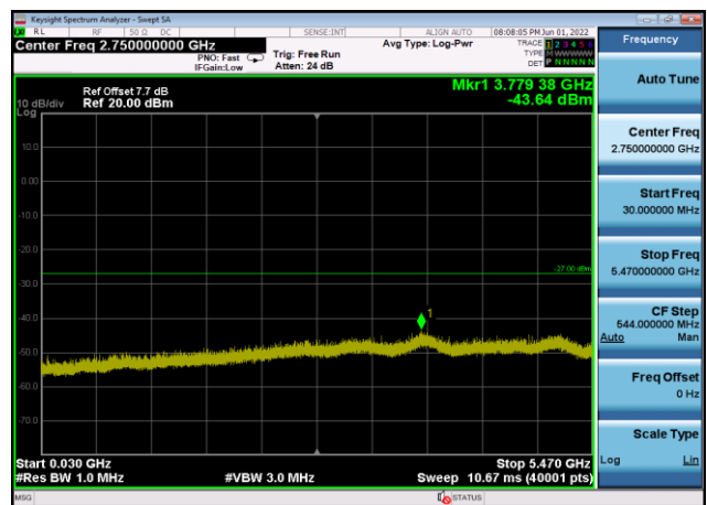
U-NII-2c ,Plot 2,30MHz~5470MHz-802.11 n(40MHz),5670MHz,Ant8
