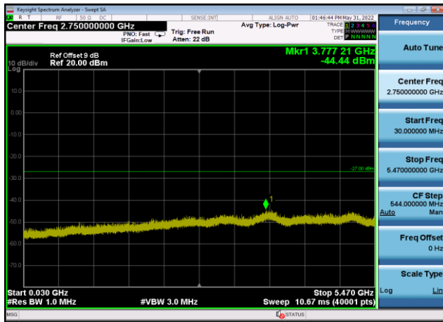
U-NII-2c ,Plot 2,30MHz~5470MHz-802.11 n(40MHz),5590MHz,Ant9
