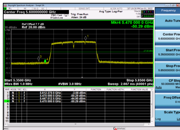
U-NII-2c ,Plot 1,Band Edge-802.11ac(2 0MHz),5500MHz,Ant8
