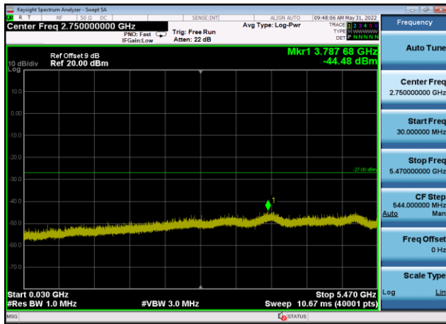
U-NII-2c ,Plot 2,30MHz~5470MHz-802.11 n(20MHz),5600MHz,Ant9
