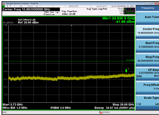
U-NII-2c ,Plot 3,5725MHz~26000MHz-802 .11n(40MHz),5590MHz,Ant9
