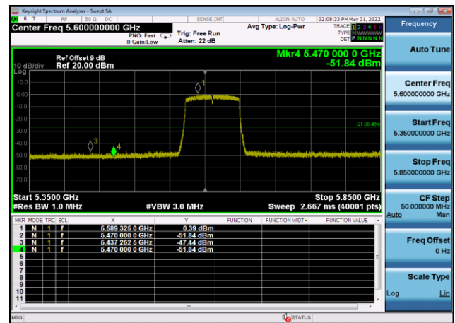
U-NII-2c ,Plot 1,Band Edge-802.11ax(1 60MHz),5570MHz,Ant9
