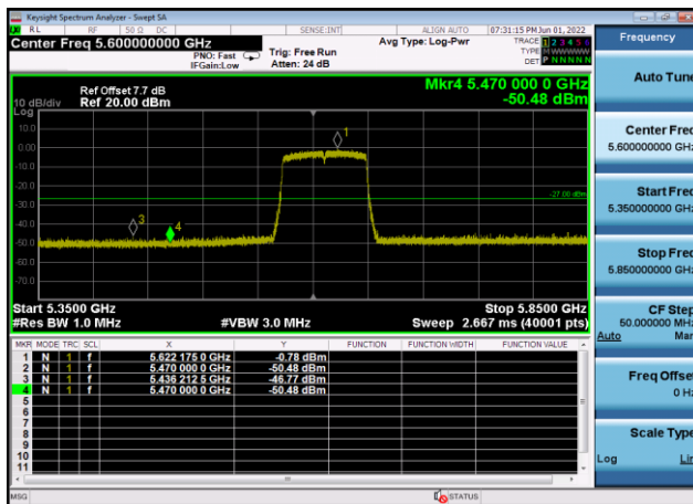
U-NII-2c ,Plot 1,Band Edge-802.11ac(8 0MHz),5610MHz,Ant8
