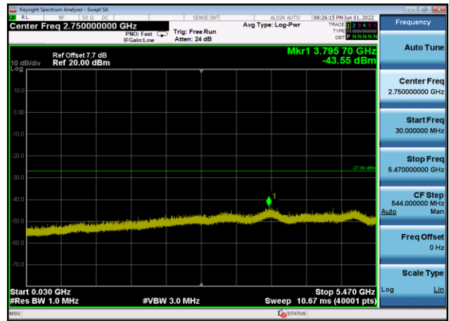
U-NII-2c ,Plot 2,30MHz~5470MHz-802.11 n(20MHz),5600MHz,Ant8
