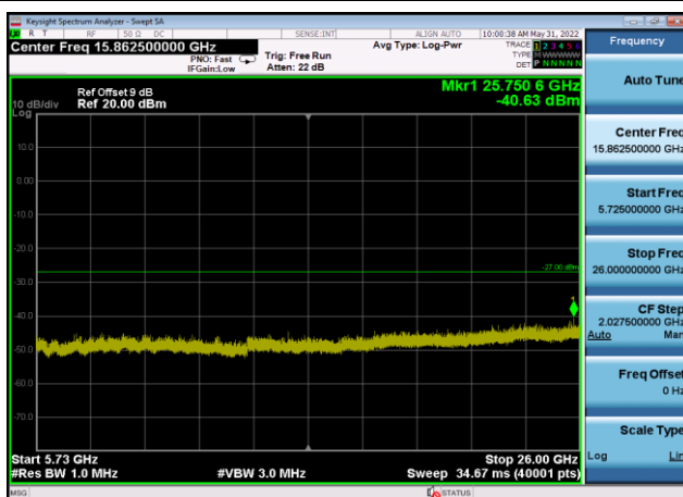
U-NII-2c ,Plot 3,5725MHz~26000MHz-802 .11n(20MHz),5700MHz,Ant9
