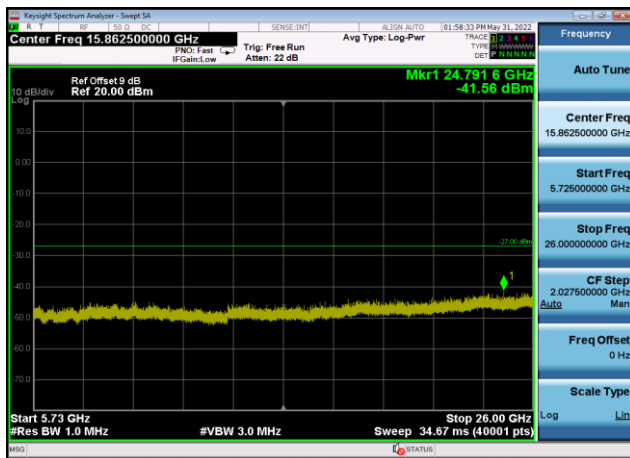
U-NII-2c ,Plot 3,5725MHz~26000MHz-802 .11n(40MHz),5670MHz,Ant9
