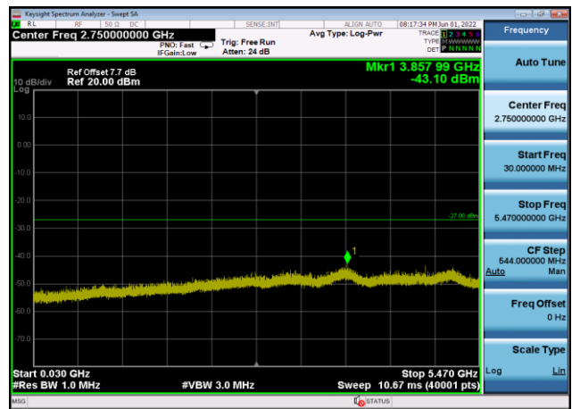
U-NII-2c ,Plot 2,30MHz~5470MHz-802.11 n(20MHz),5700MHz,Ant8
