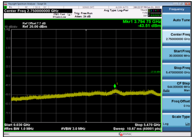
U-NII-2c ,Plot 2,30MHz~5470MHz-802.11 n(20MHz),5700MHz,Ant8
