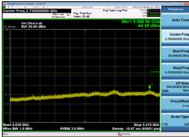
U-NII-2c ,Plot 2,30MHz~5470MHz-802.11 n(20MHz),5700MHz,Ant9
