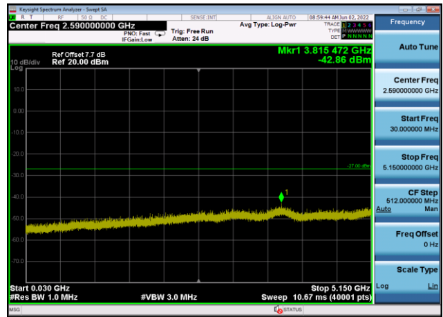
U-NII-1 ,Plot 2,30MHz~5150MHz-802.11n (20MHz),5220MHz,Ant8
