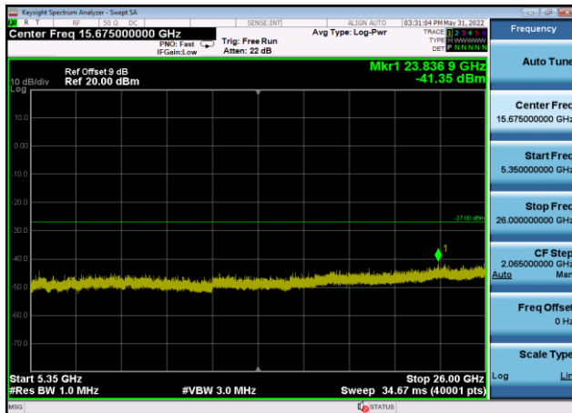
U-NII-1 ,Plot 3,5350MHz~26000MHz-802. 11n(20MHz),5220MHz,Ant9
