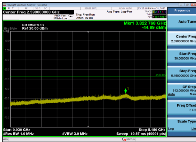
U-NII-1 ,Plot 2,30MHz~5150MHz-802.11n (20MHz),5240MHz,Ant9
