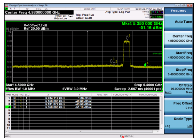
U-NII-1 ,Plot 1,Band Edge-802.11ac(80 MHz),5210MHz,Ant8
