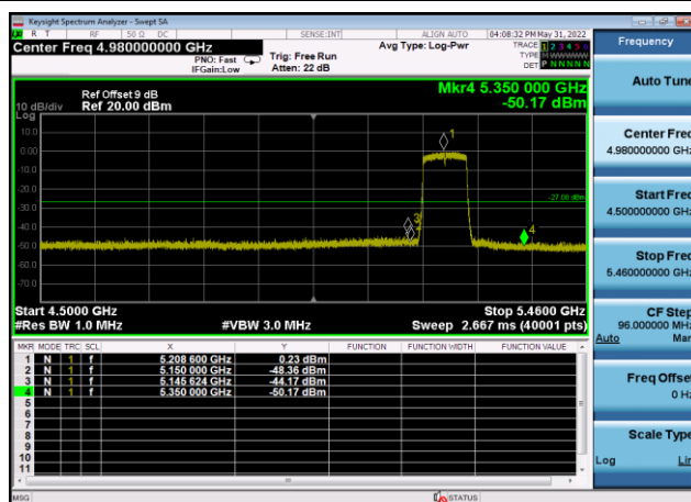
U-NII-1 ,Plot 1,Band Edge-802.11ac(80 MHz),5210MHz,Ant9
