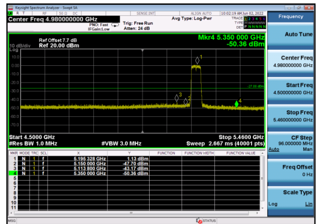
U-NII-1 ,Plot 1,Band Edge-802.11ac(40 MHz),5230MHz,Ant8
