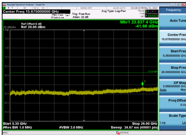
U-NII-1 ,Plot 3,5350MHz~26000MHz-802. 11n(20MHz),5240MHz,Ant9
