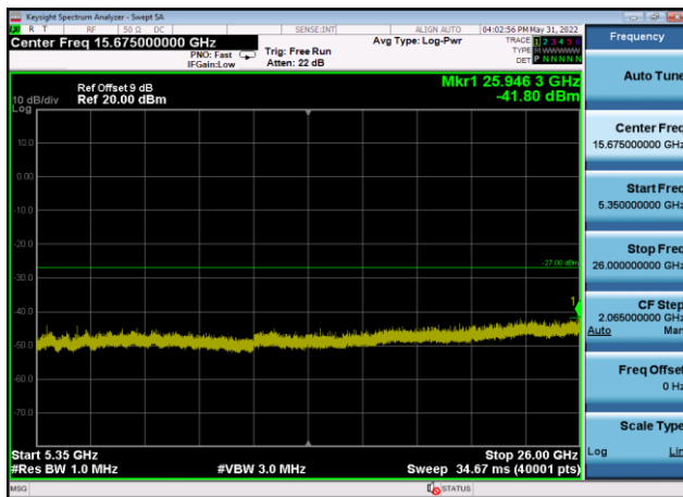
U-NII-1 ,Plot 3,5350MHz~26000MHz-802.11n(40MHz),5230MHz,Ant9
