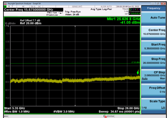
U-NII-1 ,Plot 3,5350MHz~26000MHz-802. 11n(20MHz),5220MHz,Ant8
