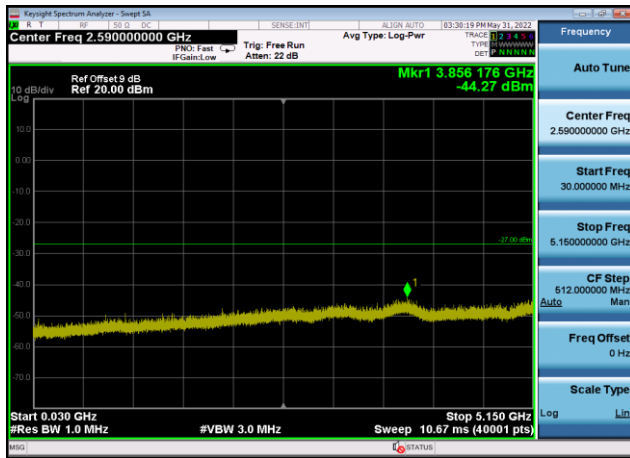
U-NII-1 ,Plot 2,30MHz~5150MHz-802.11n (20MHz),5220MHz,Ant9
