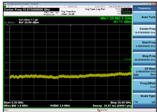
U-NII-1 ,Plot 3,5350MHz~26000MHz-802. 11n(20MHz),5240MHz,Ant8
