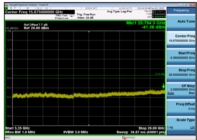
U-NII-1 ,Plot 3,5350MHz~26000MHz-802.11n(40MHz),5230MHz,Ant8
