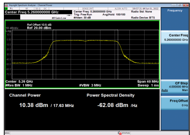
U-NII-2a Output Power-802.11ac(20MHz) ,5260MHz,Ant8
