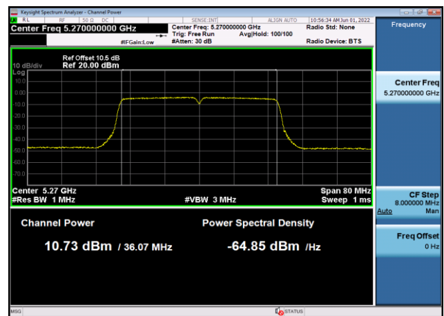
U-NII-2a Output Power-802.11ac(40MHz) ,5270MHz,Ant8
