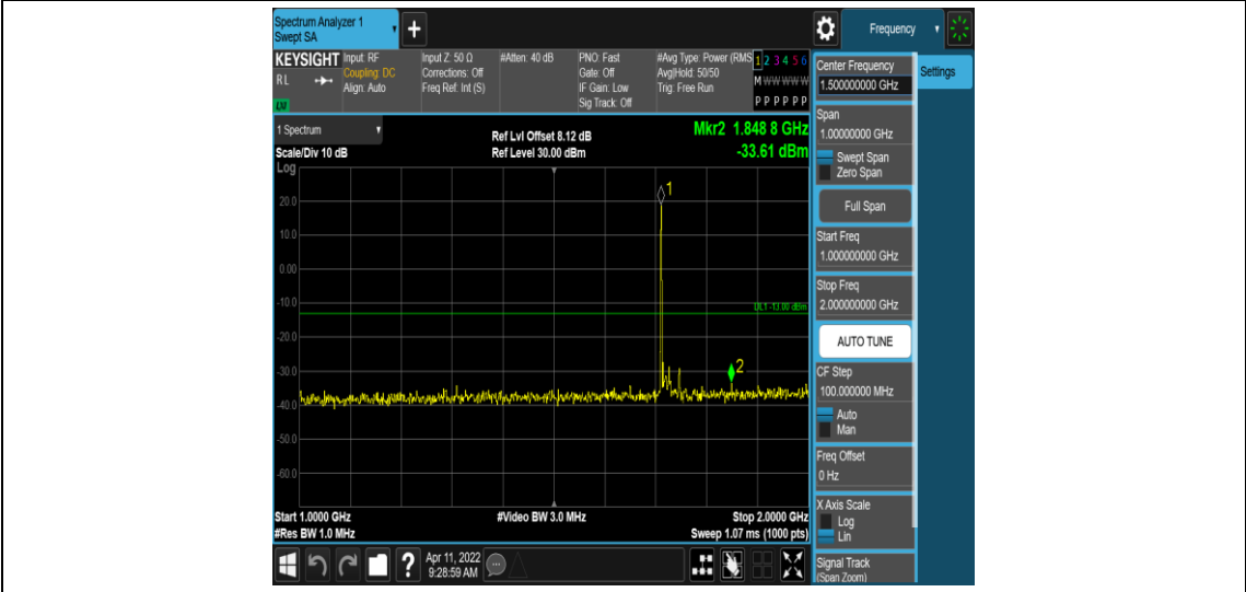
Band4-20MHz-QPSK-20050-1RB#0-Range4:1000~2000MHz
