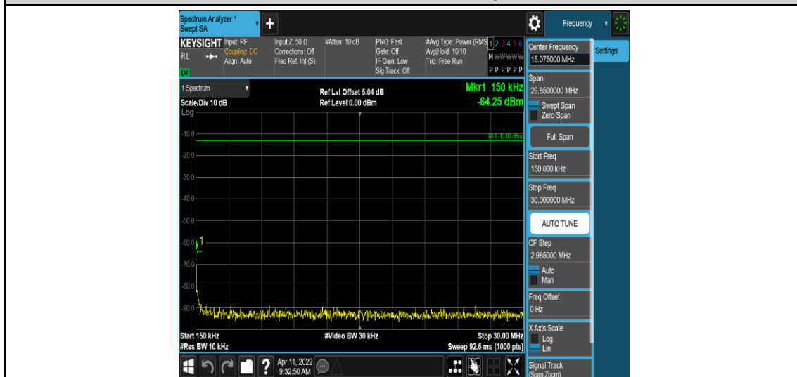
Band4-20MHz-QPSK-20300-1RB#0-Range2:0.15~30MHz
