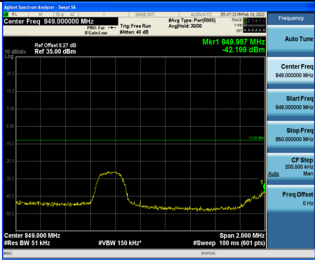
Band5-3MHz-QPSK-20635-1RB#14
