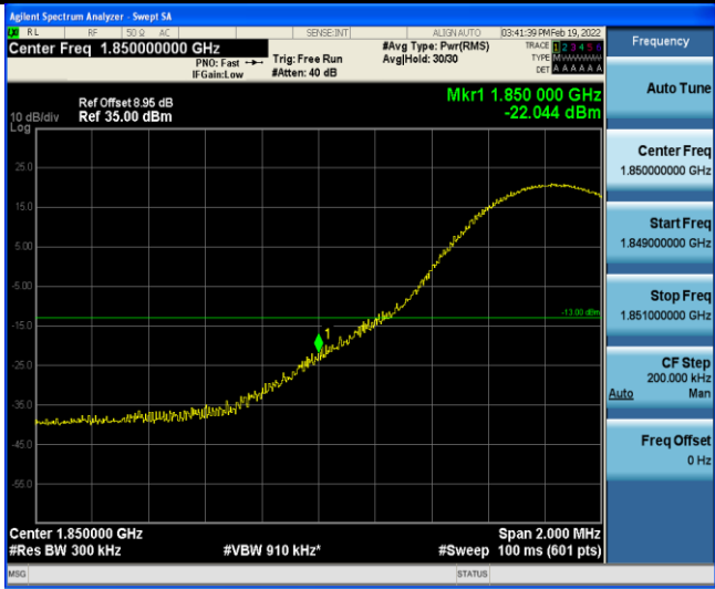
Band2-15MHz-16QAM-18675-1RB#74
