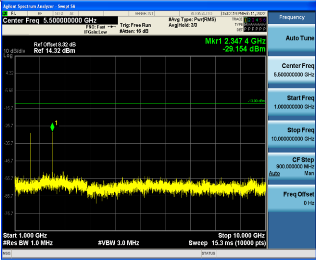
Band13-5MHz-QPSK-23255-1RB#0-Range4:1000~10000MHz
