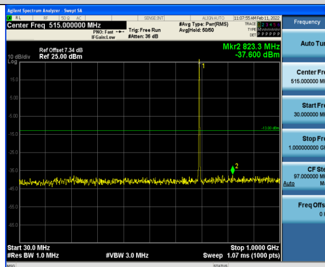
Band12-1.4MHz-QPSK-23017-1RB#0-Range3:30~1000MHz
