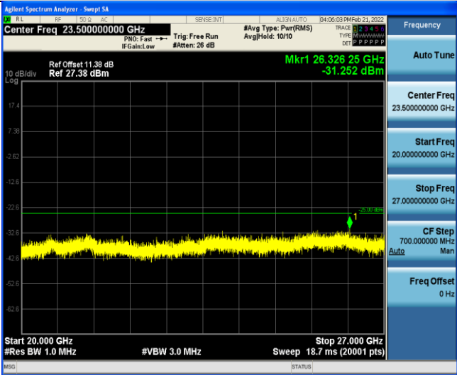
Band7-20MHz-QPSK-20850-1RB#0-Range3:20000~27000MHz
