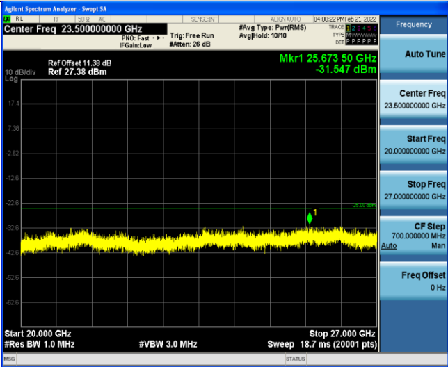
Band7-20MHz-QPSK-21100-1RB#0-Range3:20000~27000MHz
