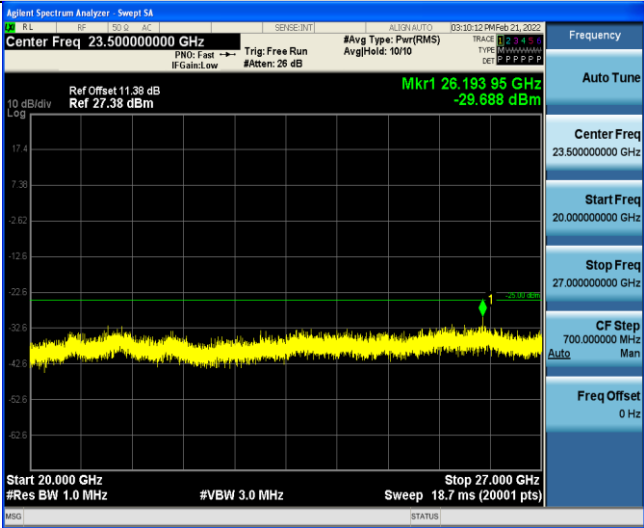
Band7-15MHz-QPSK-20825-1RB#0-Range5:20000~27000MHz
