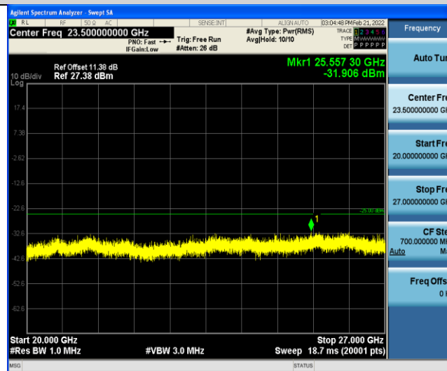
Band7-5MHz-QPSK-21425-1RB#0-Range5:20000~27000MHz
