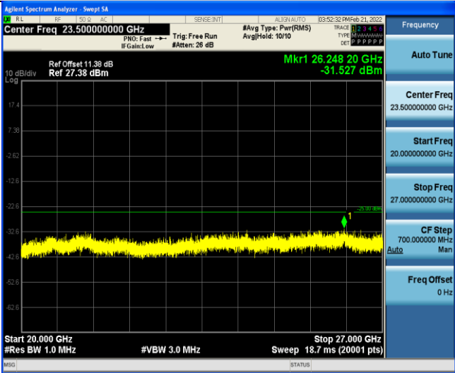
Band7-10MHz-QPSK-21400-1RB#0-Range3:20000~27000MHz
