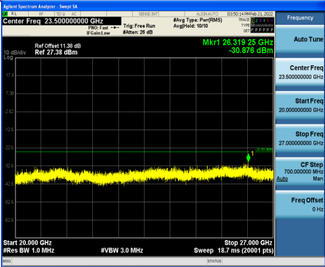
Band7-10MHz-QPSK-21100-1RB#0-Range3:20000~27000MHz
