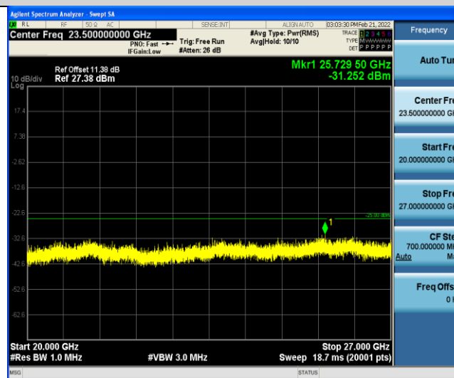
Band7-5MHz-QPSK-21100-1RB#0-Range5:20000~27000MHz
