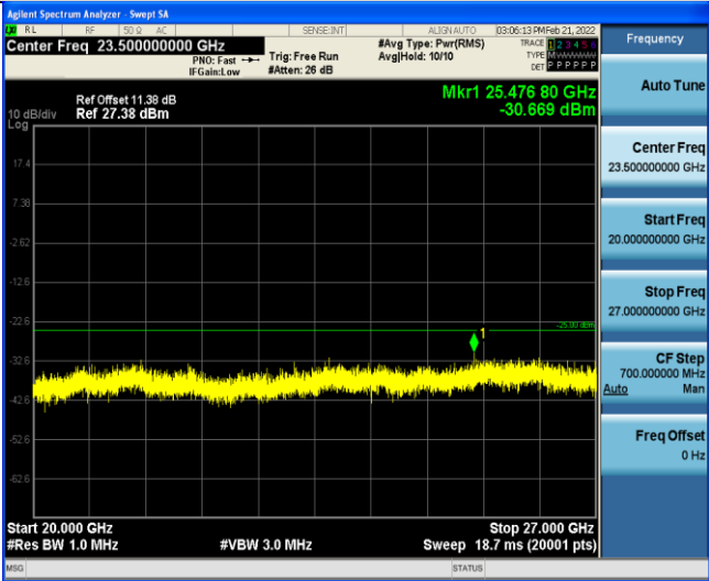
Band7-10MHz-QPSK-20800-1RB#0-Range5:20000~27000MHz
