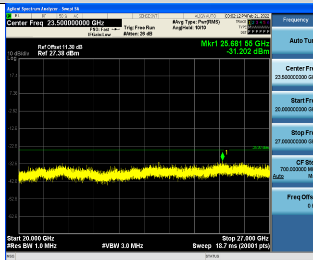
Band7-5MHz-QPSK-20775-1RB#0-Range5:20000~27000MHz
