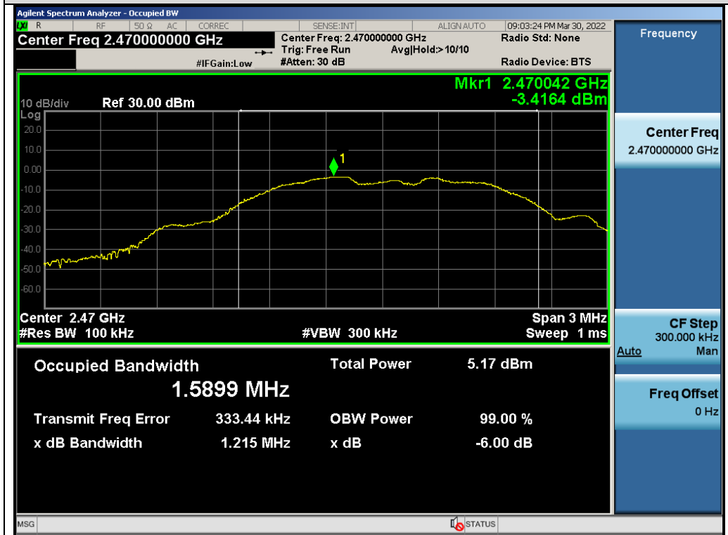
Test_Graph_GFSK_ANT1_2470_DTSBW
