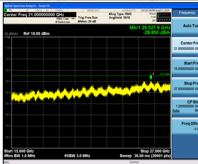
Band7-20MHz-QPSK-21100-1RB#0-Range3:15000~27000MHz
