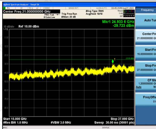
Band7-10MHz-QPSK-21400-1RB#0-Range3:15000~27000MHz
