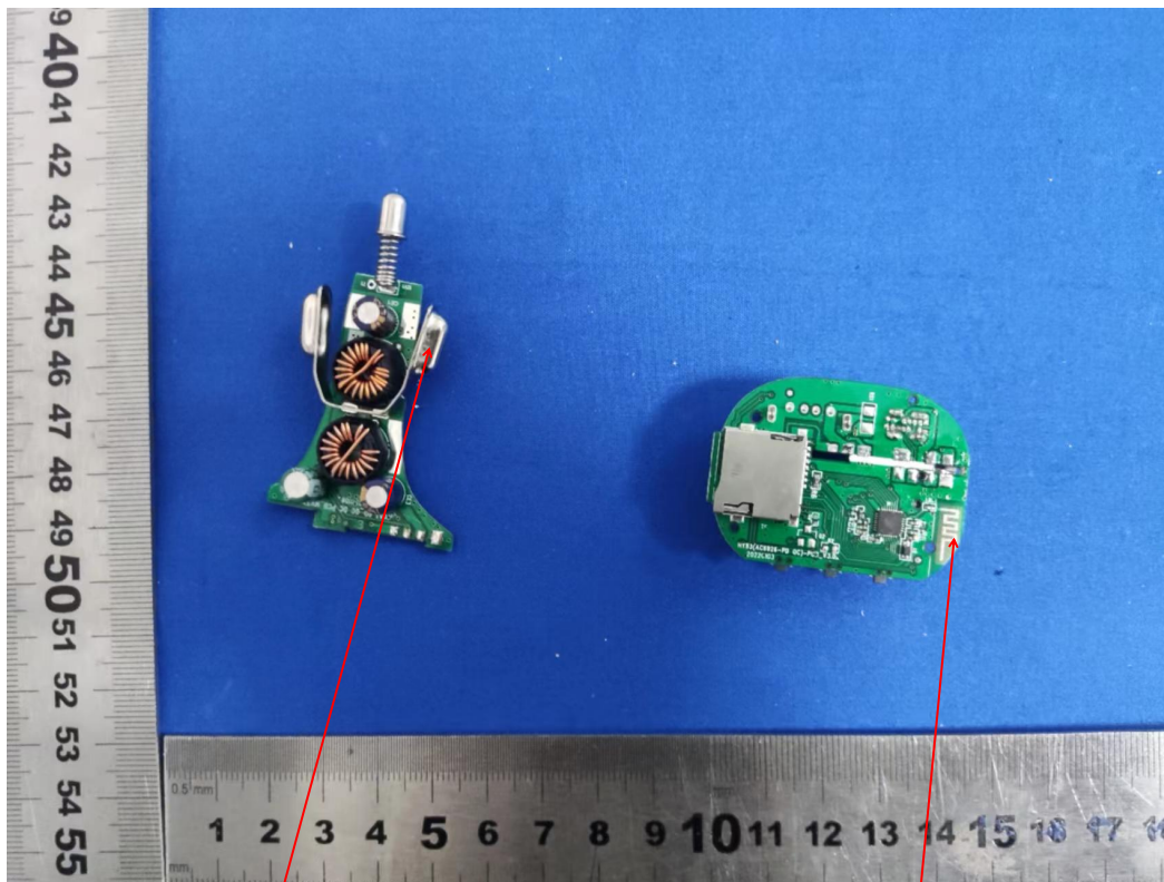
FM ANT
