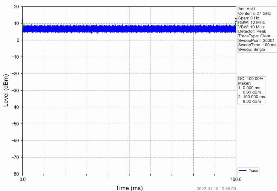
802.11ac(VHT40)_LCH_5270MHz_Ant1_NTNV
