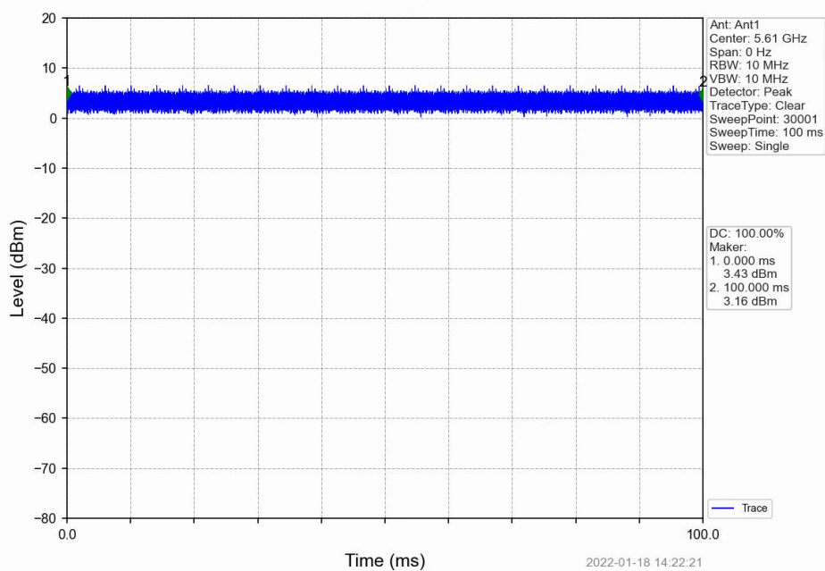
802.11ac(VHT80)_HCH_5610MHz_Ant1_NTNV
