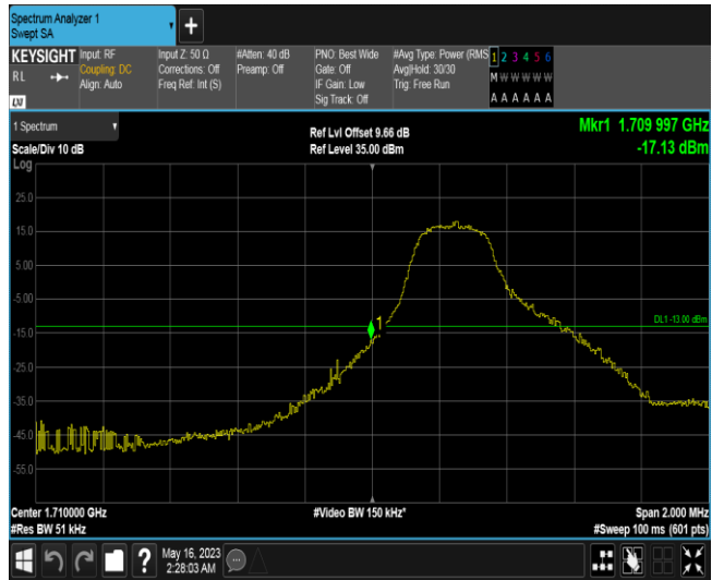
Band4-3MHz-QPSK-19965-1RB#14
