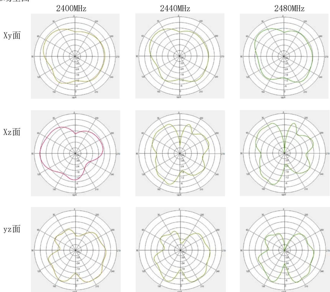
2D场型图
