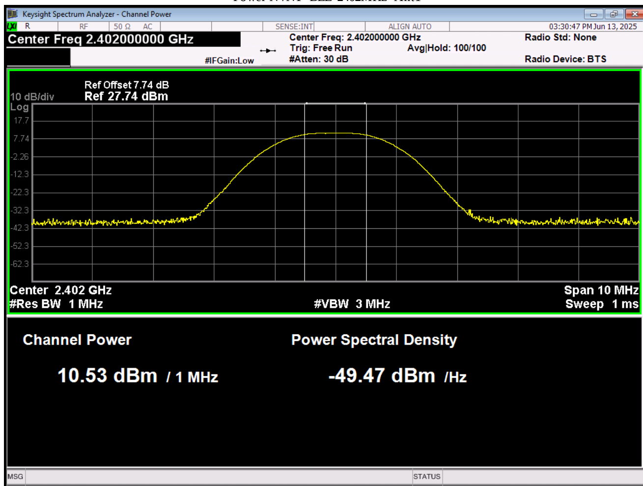
Power NVNT BLE 2402MHz Ant1
