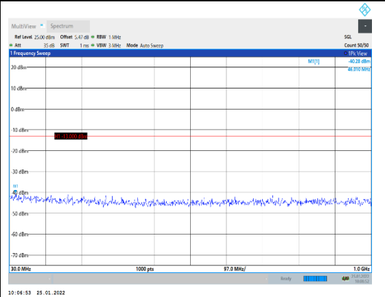
Band2-5MHz-16QAM-19175-1RB#0-Range1:3 300~1000MHz
