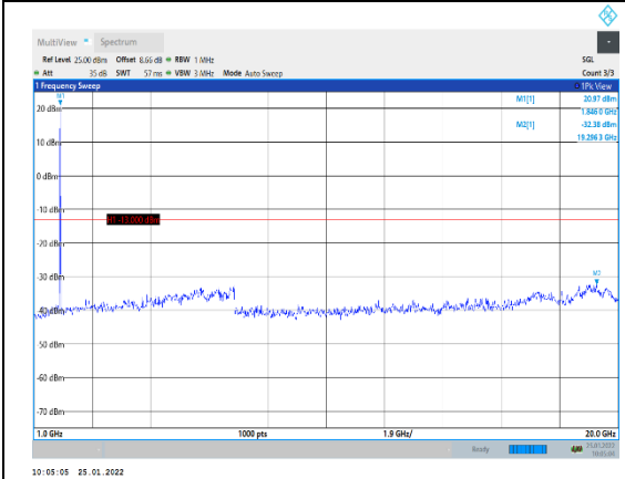
Band2-5MHz-16QAM-18625-1RB#0-Range2: 000~20000MHz
