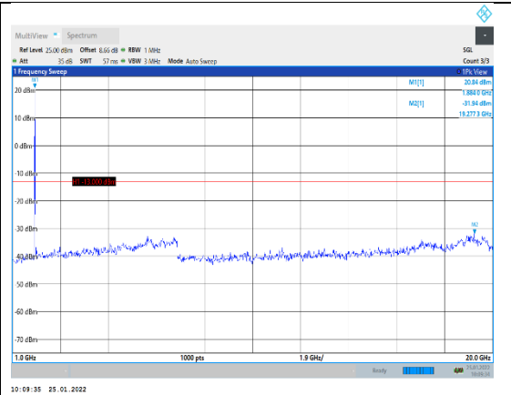
Band2-10MHz-16QAM-18900-1RB#0-Range2: 1000~20000MHz
