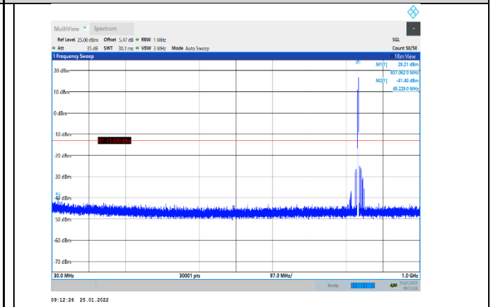
GPRS850-251-3-30~1000MHz
