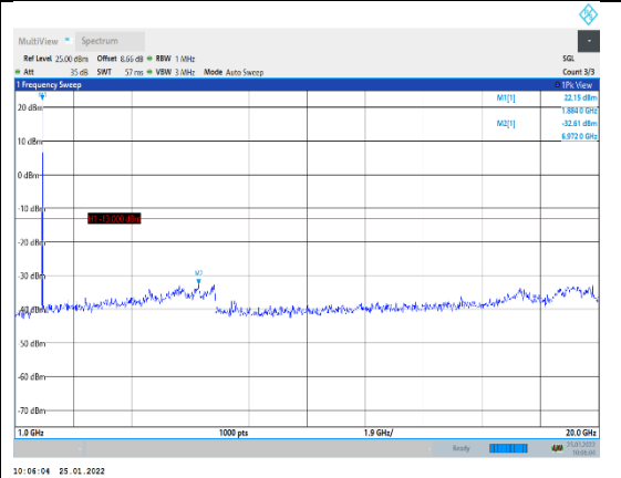
Band2-5MHz-16QAM-18900-1RB#0-Range2:1 1000~20000MHz
