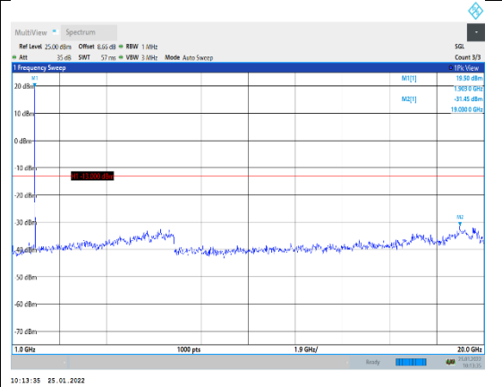
Band2-15MHz-QPSK-19125-1RB#0-Range2:1 1000~20000MHz
