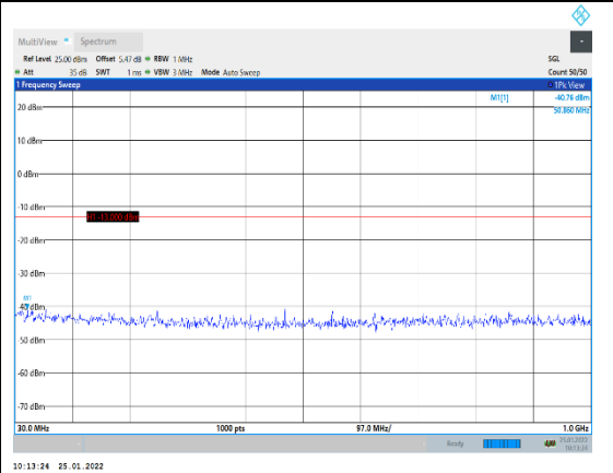
Band2-15MHz-QPSK-19125-1RB#0-Range1:3 0~1000MHz
