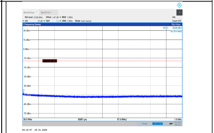
GSM1900-810-0-30~1000MHz
