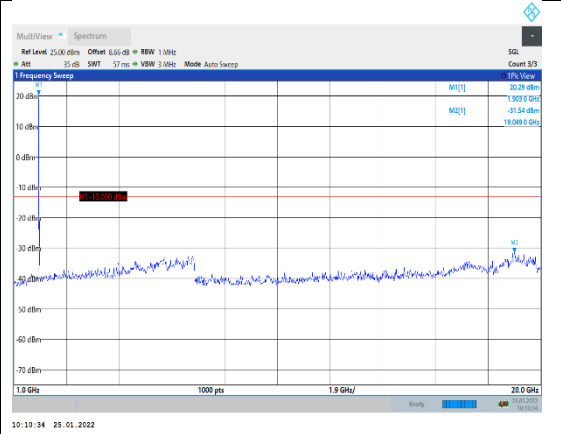
Band2-10MHz-16QAM-19150-1RB#0-Range2: 1000~20000MHz
