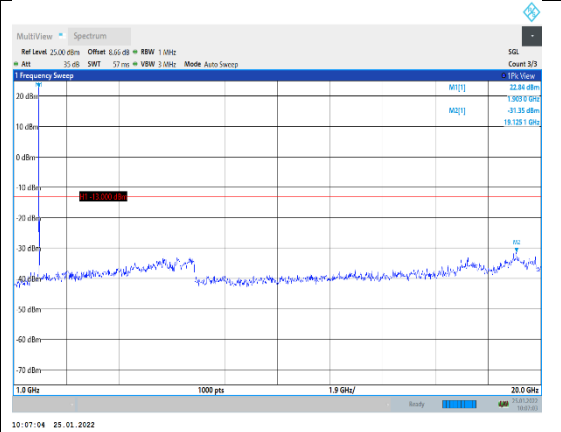
Band2-5MHz-16QAM-19175-1RB#0-Range2:1 1000~20000MHz
