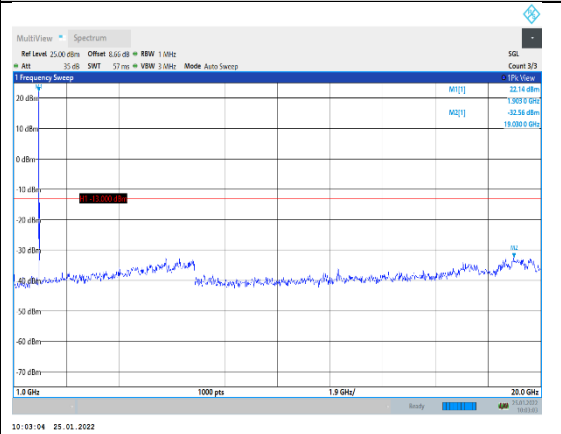
Band2-3MHz-QPSK-19185-1RB#0-Range 2:10 00~20000MHz
