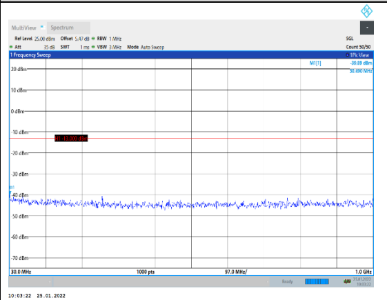
Band2-3MHz-16QAM-19185-1RB#0-Range1:3 0~1000MHz
