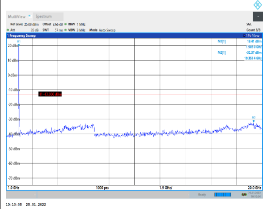
Band2-10MHz-QPSK-19150-1RB#0-Range2:1 000~20000MHz
