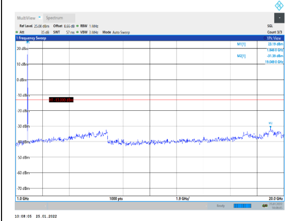
Band2-10MHz-QPSK-18650-1RB#0-Range2: 000~20000MHz
