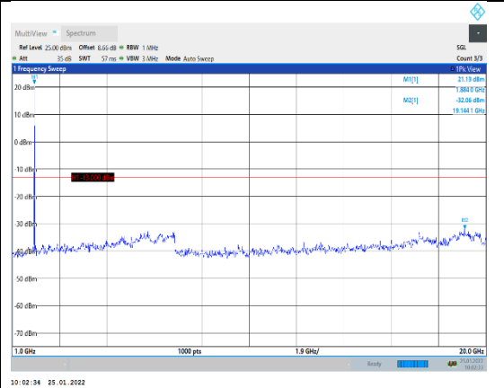
Band2-3MHz-16QAM-18900-1RB#0-Range2:1 000~20000MHz
