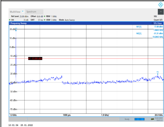
Band2-3MHz-16QAM-18615-1RB#0-Range2: 000~20000MHz
