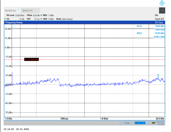
Band2-15MHz-16QAM-19125-1RB#0-Range2: 1000~20000MHz
