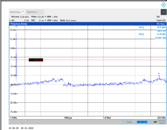
Band2-5MHz-QPSK-18625-1RB#0-Range 2:1 00~20000MHz
