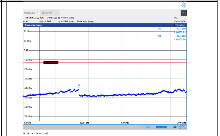
EGPRS1900-810-2-1000~20000MHz
