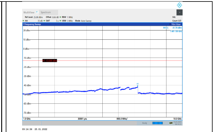
EGPRS850-190-8-1000~10000MHz
