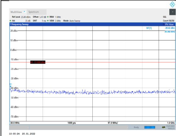
Band2-5MHz-QPSK-18900-1RB#0-Range 1:3 ~1000MHz
