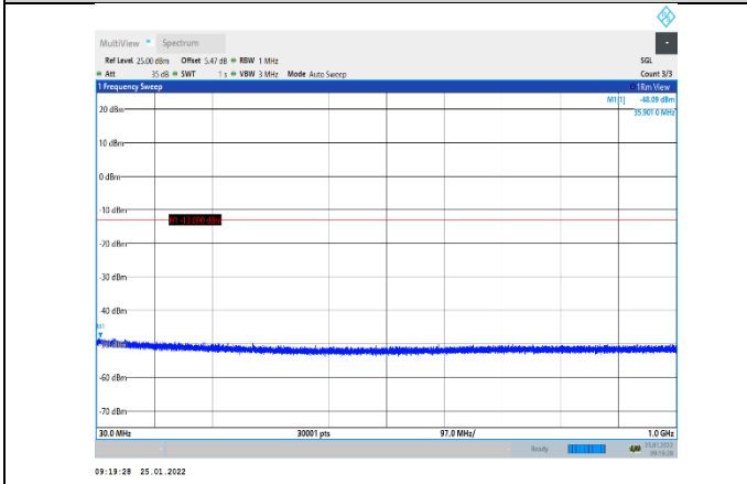
GSM1900-661-0-30~1000MHz
