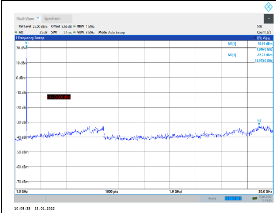
Band2-10MHz-16QAM-18650-1RB#0-Range2: 1000~20000MHz
