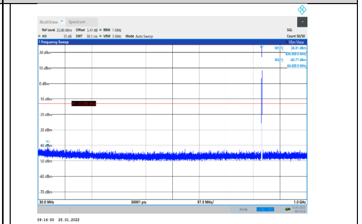
EGPRS850-251-8-30~1000MHz
