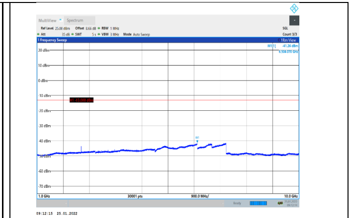
GPRS850-190-3-1000~10000MHz
