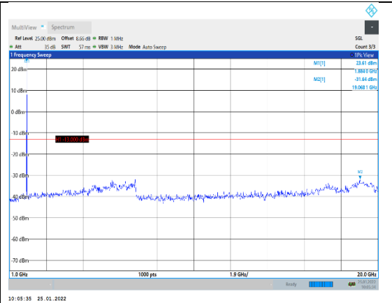
Band2-5MHz-QPSK-18900-1RB#0-Range 2:10 00~20000MHz
