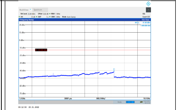
GPRS850-251-3-1000~10000MHz
