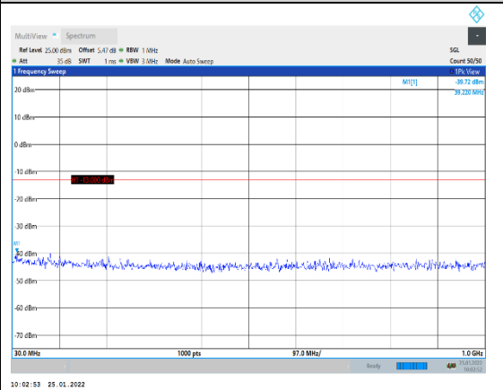
Band2-3MHz-QPSK-19185-1RB#0-Range 1:30 ~1000MHz
