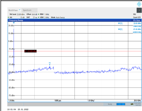
Band2-3MHz-QPSK-18615-1RB#0-Range 2:1 00~20000MHz
