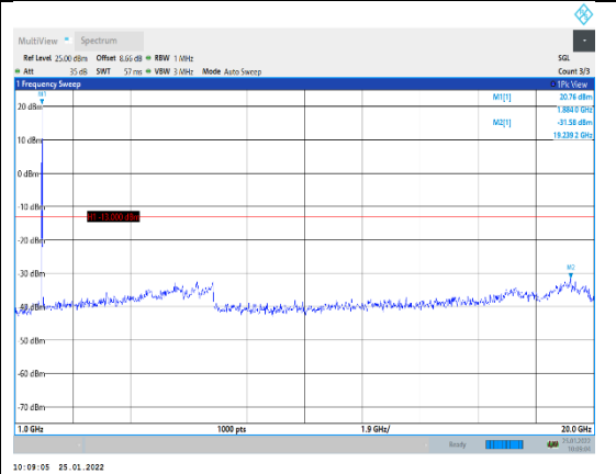
Band2-10MHz-QPSK-18900-1RB#0-Range2:1 000~20000MHz
