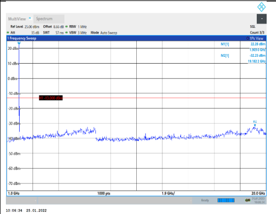
Band2-5MHz-QPSK-19175-1RB#0-Range 2:10 00~20000MHz
