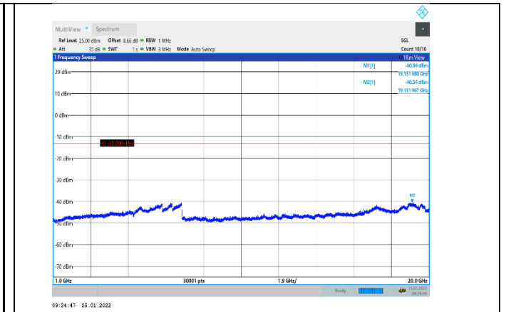
EGPRS1900-661-2-1000~20000MHz
