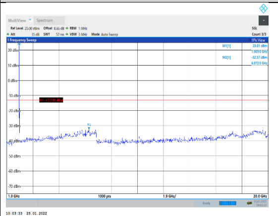
Band2-3MHz-16QAM-19185-1RB#0-Range2:1 000~20000MHz
