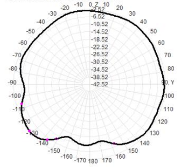
2400.0MHz Total(E2-YZ), Max=-2.52dBi
