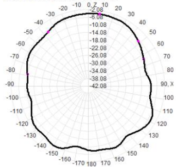
2450.0MHz Total(E1-XZ), Max=-3.97dBi
