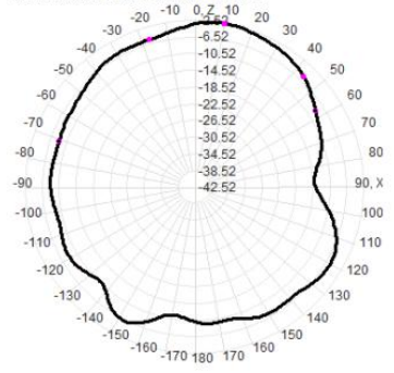
2400.0MHz Total(E1-XZ), Max=-2.65dBi
