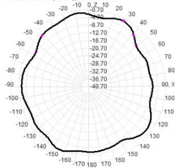
2500.0MHz Total(E1-XZ), Max=-2.18dBi
