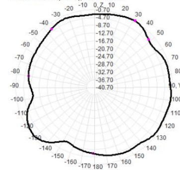
2500.0MHz Total(E2-YZ), Max=-0.70dBi
