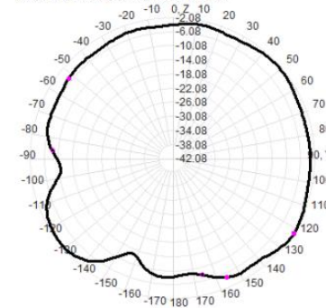
2450.0MHz Total(E2-YZ), Max=-2.08dBi
