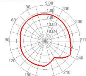
2700.000MHz H
