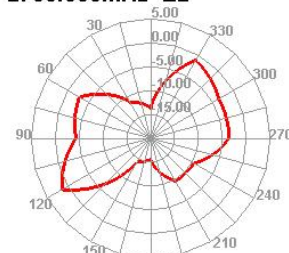
2700.000MHz E2
