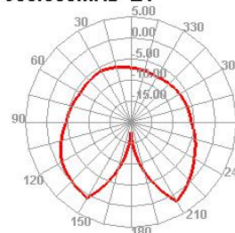
900.000MHz E1
