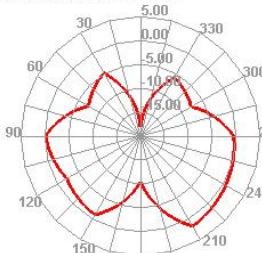
2200.000MHz E1
