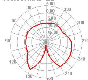
900.000MHz E2
