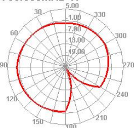
1700.000MHz H
