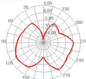
2200.000MHz E2
