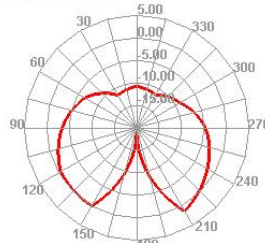
800.000MHz E1
