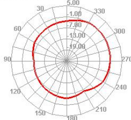
800.000MHz H
