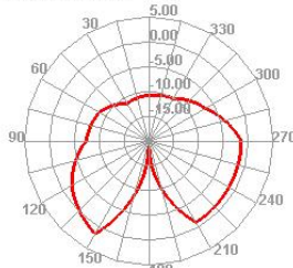
800.000MHz E2
