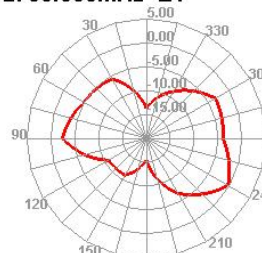
2700.000MHz E1
