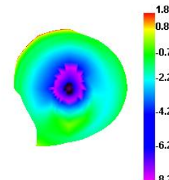
2700.000MHz E1
