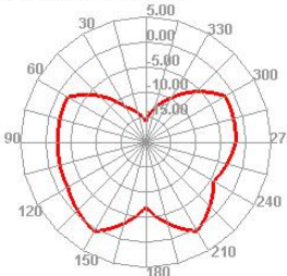
1700.000MHz E1
