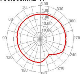
700.000MHz H
