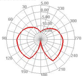
700.000MHz E1
