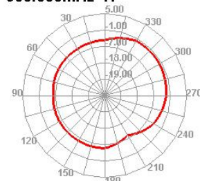
900.000MHz H
