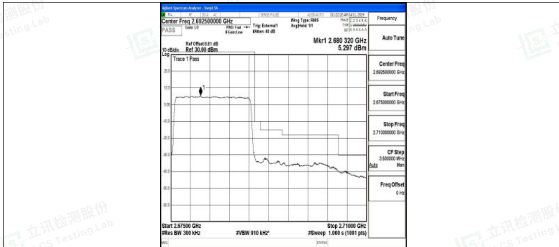
Band41_15MHz_QPSK_41515_75RB#0
