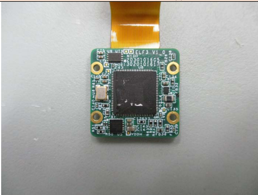
CAM MODULE_2 BOARD1 (1)
