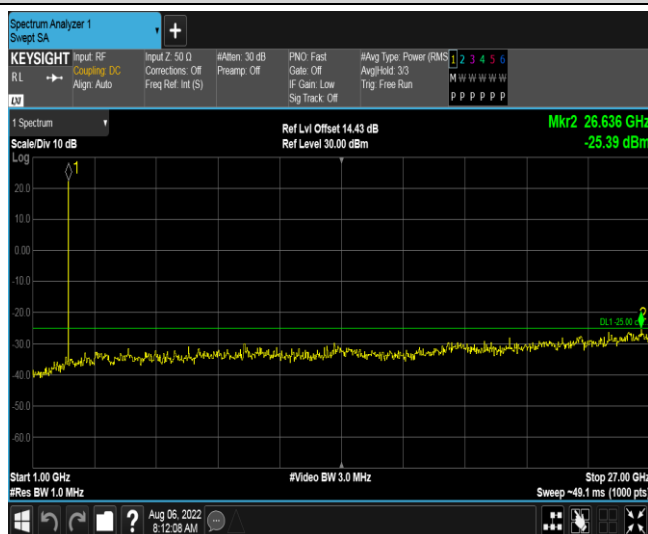
Band7-10MHz-QPSK-20800-1RB#0-Range2:1000~27000MHz
