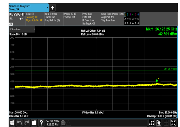
Band38-5MHz-QPSK-38000-25RB#0-20000~27000-PASS
