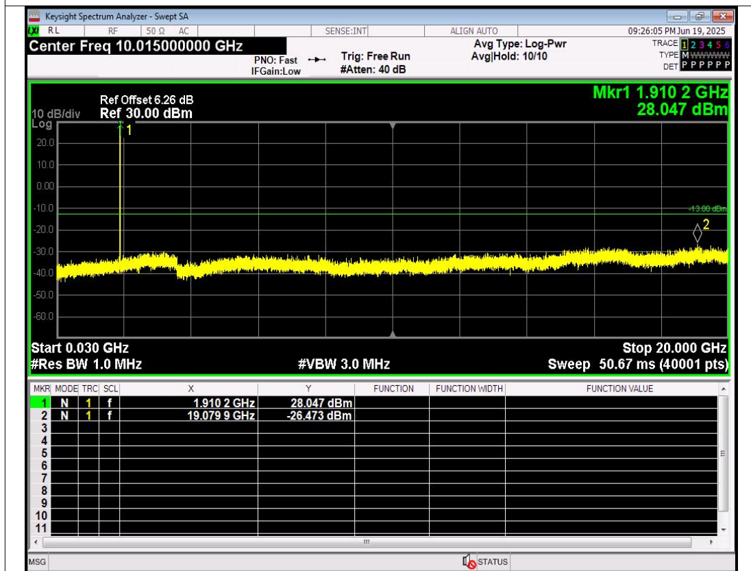
GPRS1900 Channel=810
