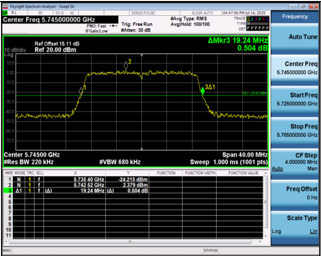
11N20MIMO-Ant1-5745
