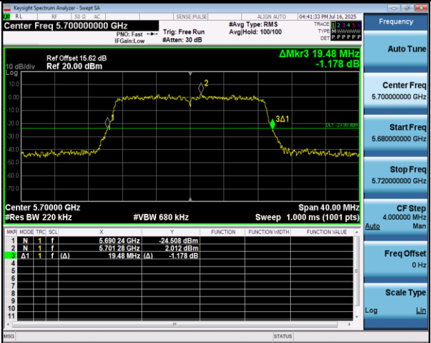
11N20MIMO-Ant2-5700
