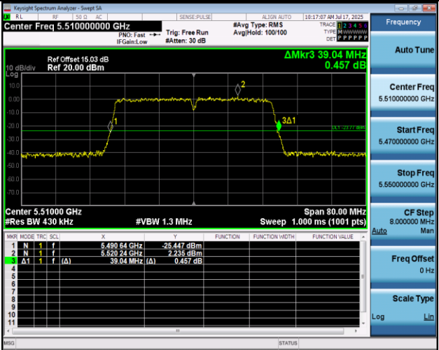
11N40MIMO-Ant1-5510
