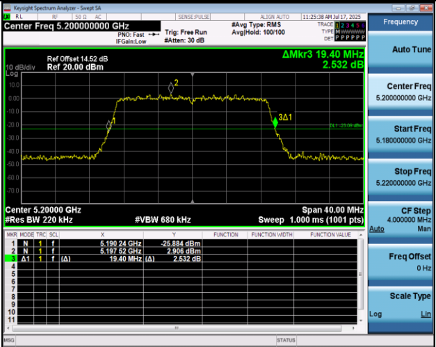
11AC20MIMO-Ant1-5200
