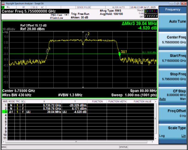
11N40MIMO-Ant1-5755
