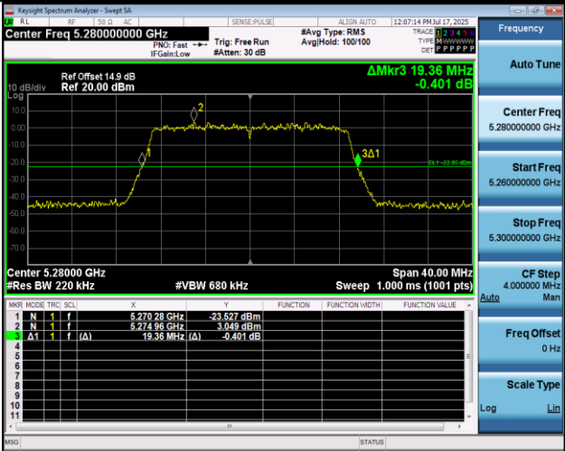
11AC20MIMO-Ant1-5280
