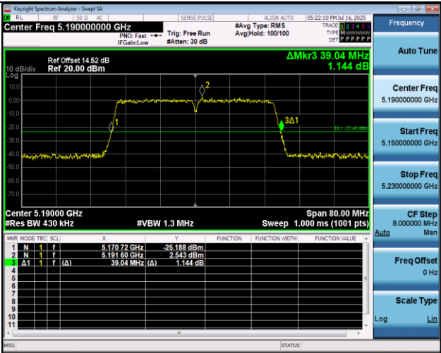
11N40MIMO-Ant1-5190
