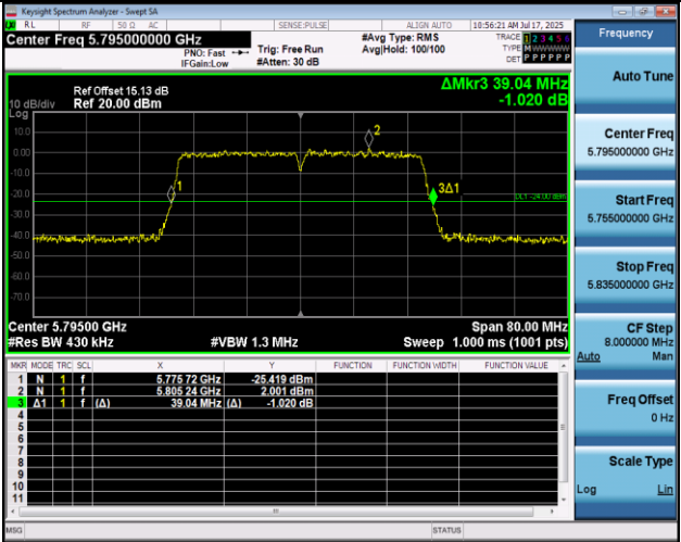
11N40MIMO-Ant1-5795
