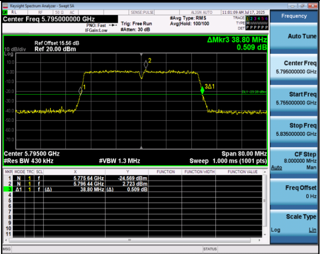
11N40MIMO-Ant2-5795
