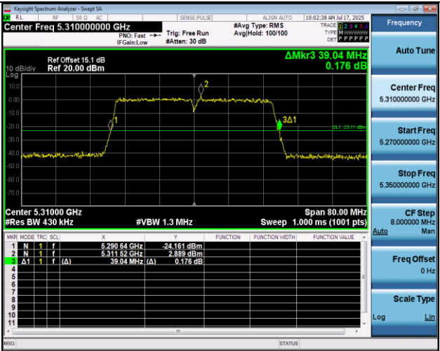
11N40MIMO-Ant1-5310
