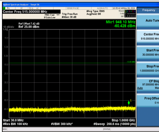
Band25-3MHz-QPSK-26675-1-0-Low-30-1000--60.43-PASS
