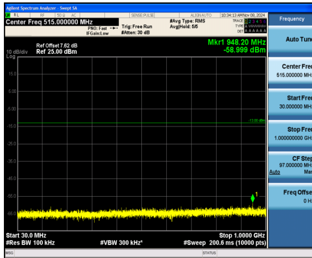
Band25-3MHz-QPSK-26365-1-0-Low-30-1000--59-PASS
