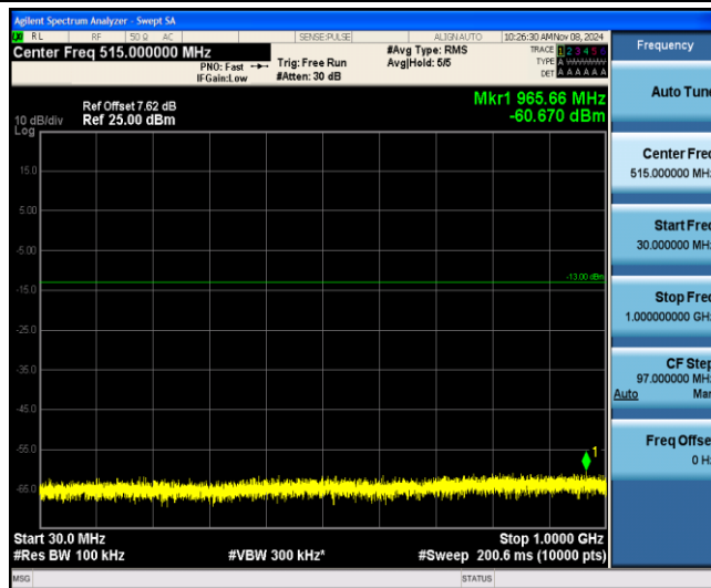
Band25-1.4MHz-QPSK-26365-1-0-Low-30-1000--60.67-PASS
