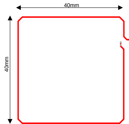
Bottom PCB layer
