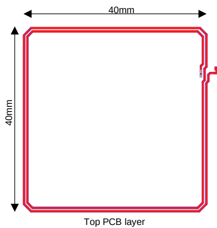
Top PCB layer
