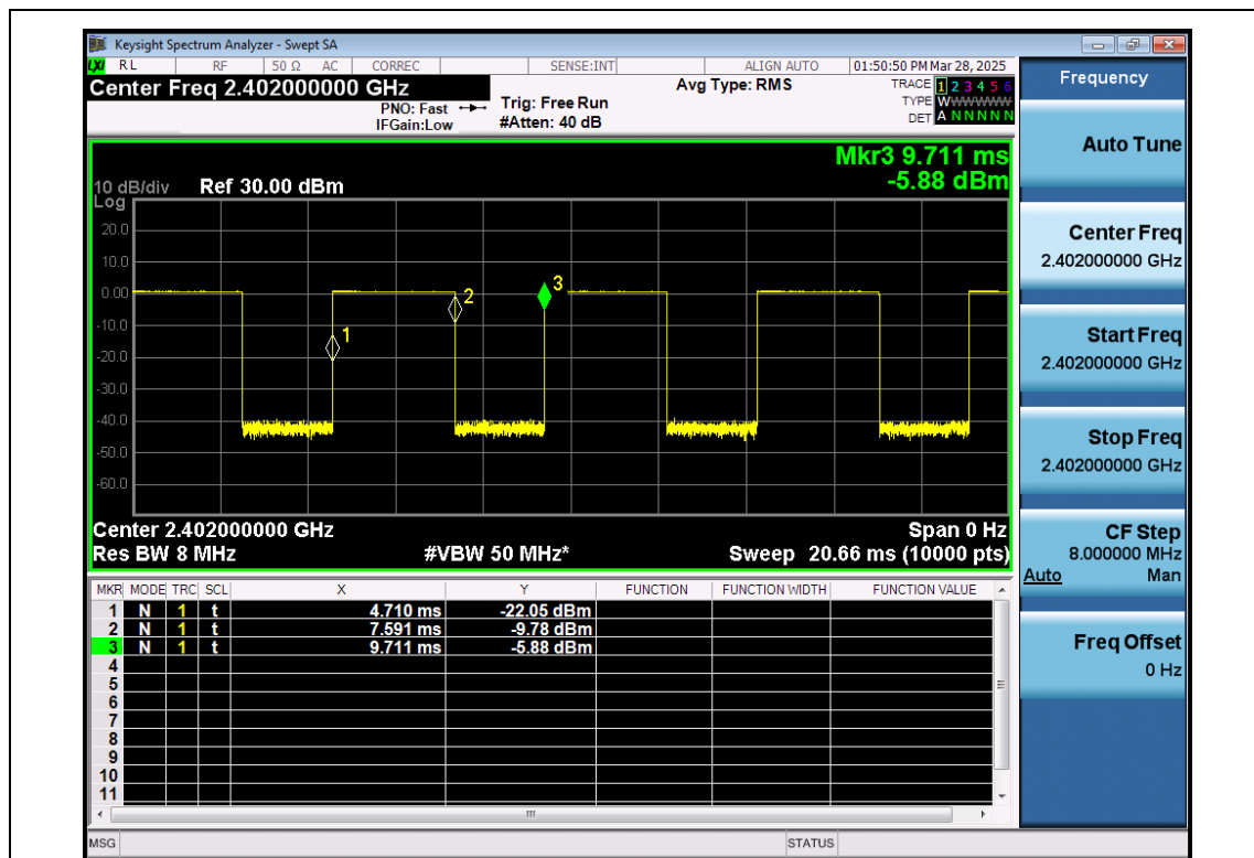
BR-GFSK-ANT1-2402
