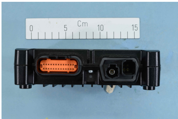
EUT Connectors
